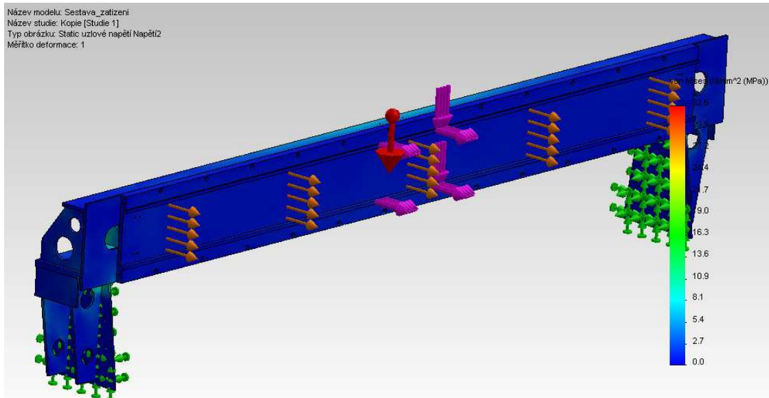
obr. 35 Zatížení příčnicku
