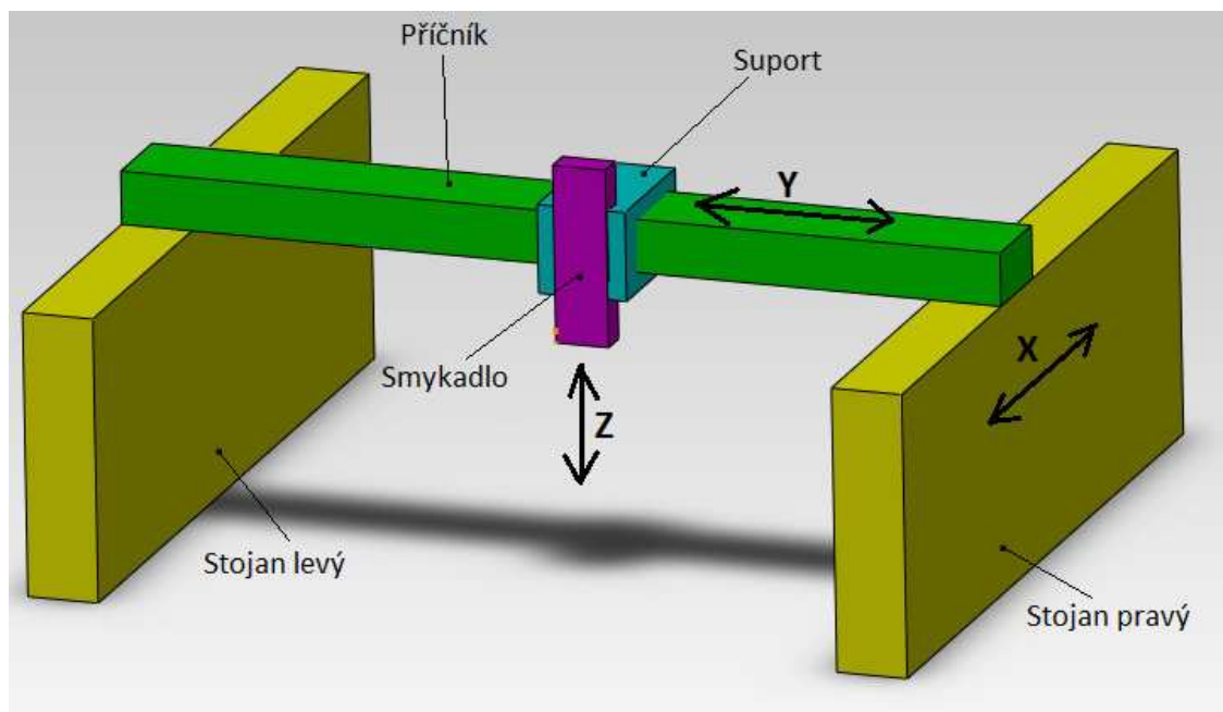
obr. 13 Horní gántry
