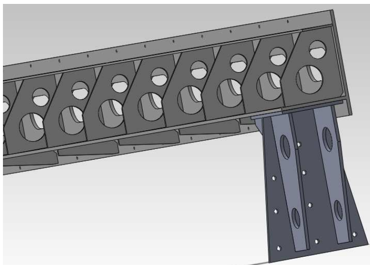
obr. 33 Příčnick s bočnicemi
