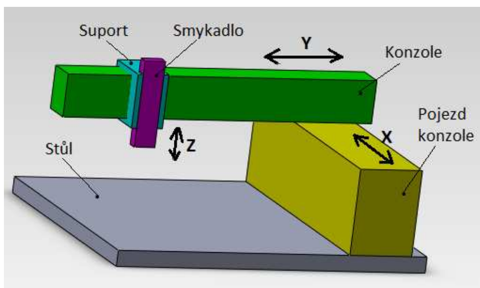
obr. 16 Konzolové provedení
