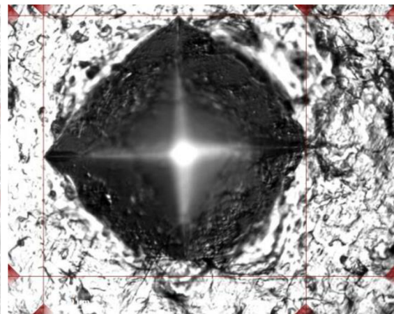
Obrázek 41: Otisk vzorku EN AW-6082 Inkubační doba: 1 [min] Tvrdost: 113.88 HV0.5
