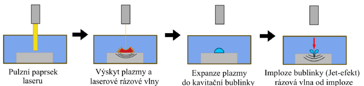
Obrázek 14: Schéma procesu laserového kavitačního zpevňování (LCP)
