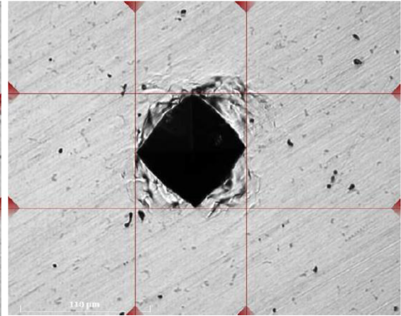
Obrázek 39: Otisk etalonu EN AW-6082 Inkubační doba: 0 [min] Tvrdost: 102.51 HV0.5
