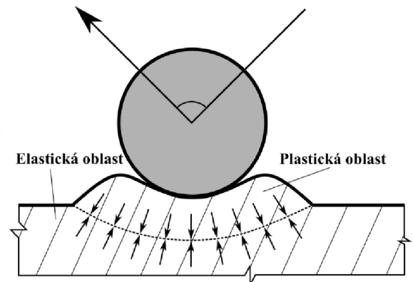
Obrázek 7: Vznik RCS na povrchu materiálu
