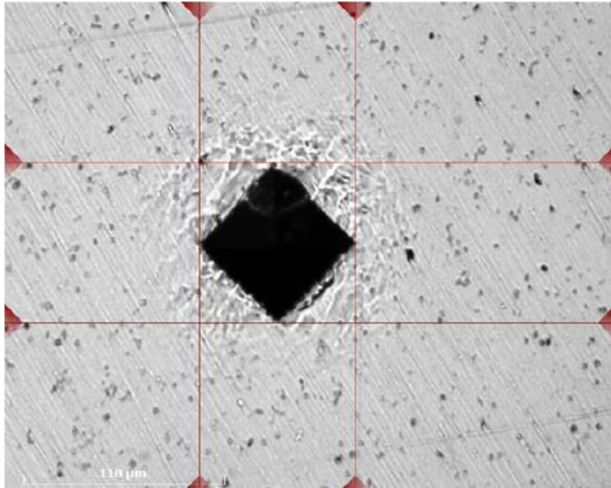
Obrázek 38: Otisk etalonu EN AW-2007 Inkubační doba: 0 [min] Tvrdost: 125.56 HV0.5
