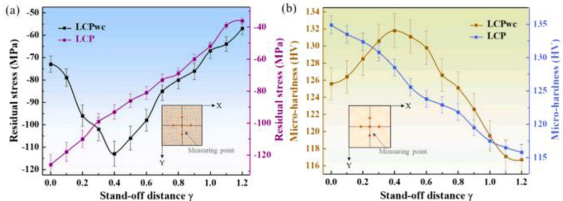
Obrázek 16: Závislost RCS a mikrotvrdosti oceli Q235 na změně vzdálenosti \gamma [21]
