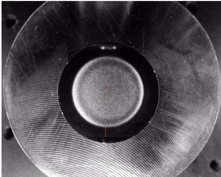
Obrázek 37: Snímek zkušební vzorku EN AW-6082 s rozvrhnutým polem vpichů
