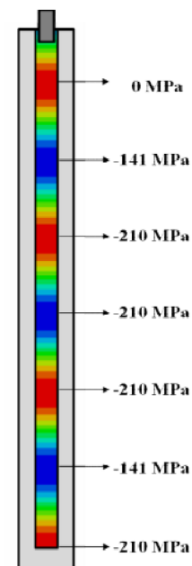
Obrázek 20: Naměřené hodnoty RCS [23]
