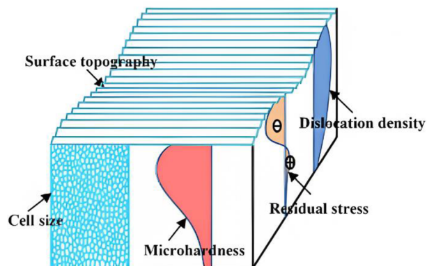
Obrázek 6: Důsledky modifikace povrchu SP [13]
