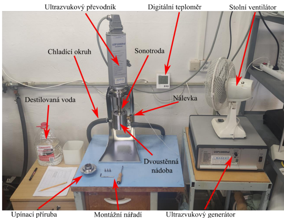
Obrázek 27: Experimentální sestava ultrazvukového kavitáčního zpevnování
