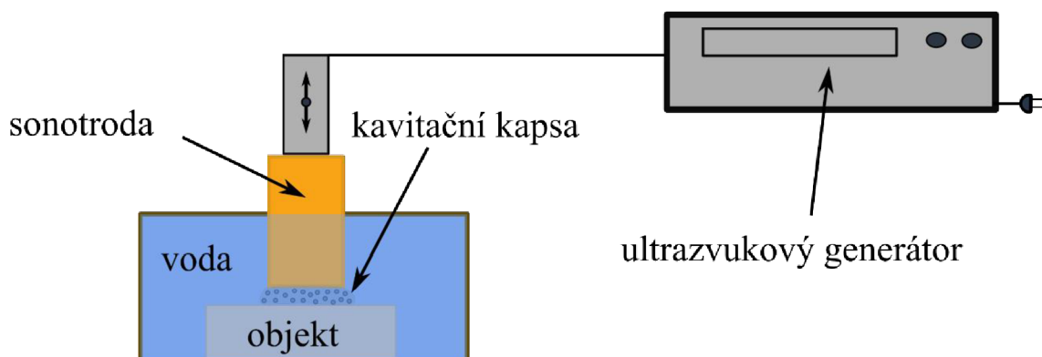
Obrázek 18: Schéma ultrazvukového kavitačního zpevňování
