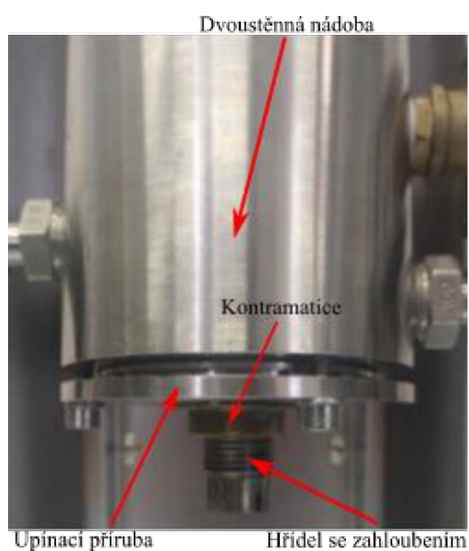
Obrázek 29: Upevnění upínací příruby do dvoustěnné nádoby
