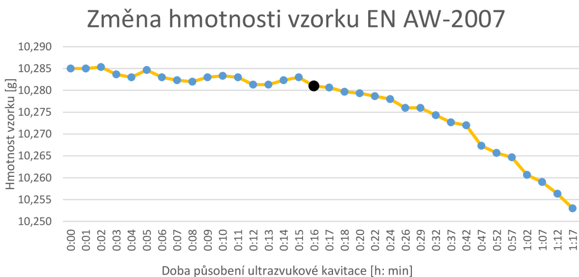
Graf 1: Změna hmotnosti vzorku EN AW-2007
