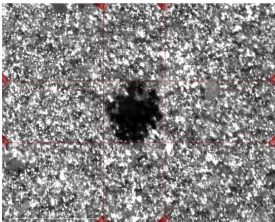
Obrázek 40: Otisk vzorku EN AW-2007 Inkubační doba: 12 [min] Tvrdost: 163.89 HV0.5
