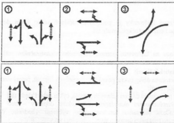
Obr. 1.2 Příklad třífázového schématu
