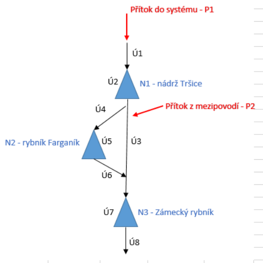
Obr. 14 Schematizace systému
