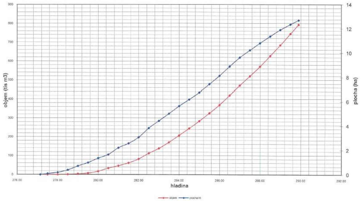
Graf 7 Batymetrické čáry nádrže Tršice [2]
