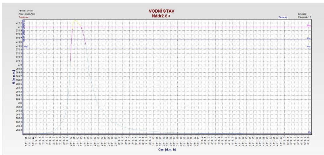
Obr. 21 Vodní stav v Zámeckém rybníku při Q_{1000} [7]
