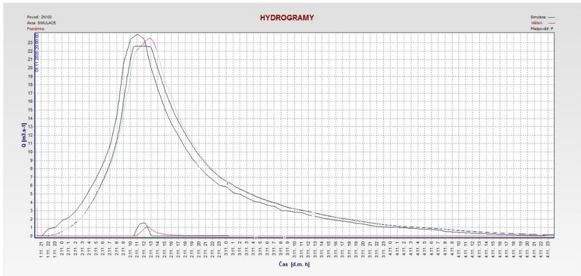
Obr. 22 Průtoky při odlehčení varianta 12 z tab. 54 [7]
