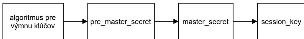
Obr. 5.1: Generovanie kľúčov
