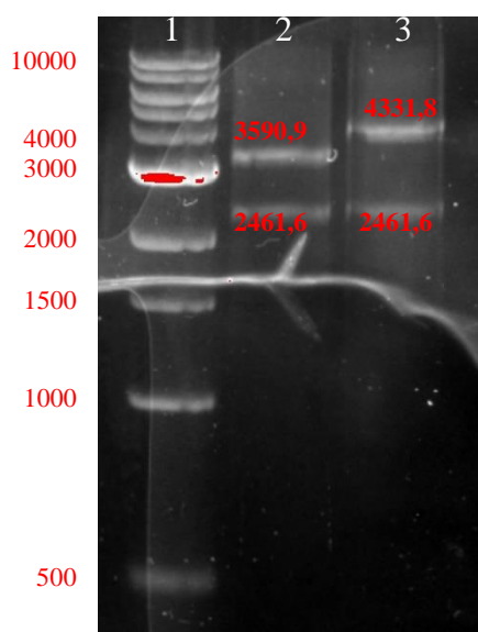
Obr. 14 Výsledek restriktivního štěpení pro ověření správnosti plasmidů obsahujících inzert. 1 - 1 kb DNA žebřík, 2 - plasmid pGEX-6P-SG Del, kolonie č. 16, 3 - plasmid pGEX-6P-SG, kolonie č. 7. Velikosti v bp uvedeny u každého fragmentu.
