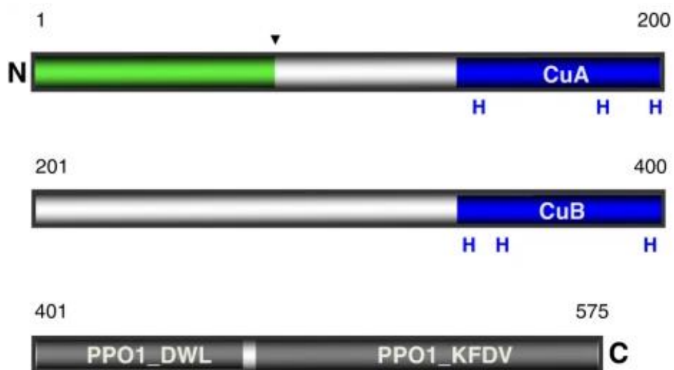
Obr. 4 Znázornění domén PPO genu. Zeleně N-terminální transítiní peptid, který je po transportu do lumen thylakoidu proteolyticky odštěpen na rozhraní s šedou částí obsahující alaninový motiv. Domény CuA a CuB s histidinovými zbytky jsou zobrazeny modře a C-terminální část šedě. Převzato a upraveno podle Tran et al. (2012).
