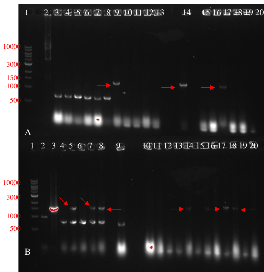
Obr. 13 Výsledek C-PCR pro ověření přítomnosti inzertu v plasmidech. A: buňky MDS42, 1 – 1 kb DNA žebřík, 2 – blank pro pPSG, 3 – pozitivní kontrola, 4-9 – pPSG (kolonie č.1-6), 10-15 – pGEX-6P-SG (kolonie 7-12), 16-21 – pGEX-6P-SG Del (kolonie č. 14-19). B: buňky TOP10, 1 – 1 kb DNA žebřík, 2 – blank pro oba pGEX, 3 – pozitivní kontrola, 4-9 – pPSG (kolonie č. 20-25), 10-15 – pGEX-6P-SG (kolonie č. 26-31), 16-21 – pGEX-6P-SG Del (kolonie č. 32-37). Červeně jsou zvýrazněny inzerty (1548 bp).
