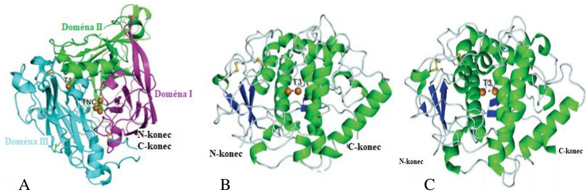
Obr. 1 Proteinové 3D struktury enzymů obsahujících jako kofaktor měď. A: Proteinová struktura lakasy izolované z kukuřice složena ze tří domén. Žlutě jsou zobrazeny disulfidické vazby. Čtyři atomy mědi jsou zobrazeny jako hnědé body. TNC označuje aktivní místo se třemi atomy kovu a T1 s jedním. B: Proteinová struktura CAT z povijnice batátové obsahující dva atomy mědi. C: Proteinová struktura aktivní formy TYR z ořešáku vlašského se stejným počtem mědi jako CAT (Převzato a upraveno podle Mydy et al. , 2021).
