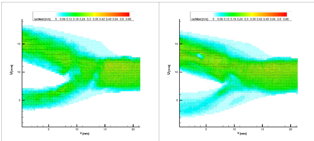
Obr. 24 Porovnání Epoxid/PDMS voda 6,267 ml/s
