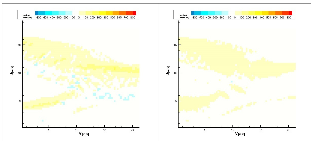
Obr. 32 Porovnání Epoxid/PDMS krevní fantom 4 ml/s
