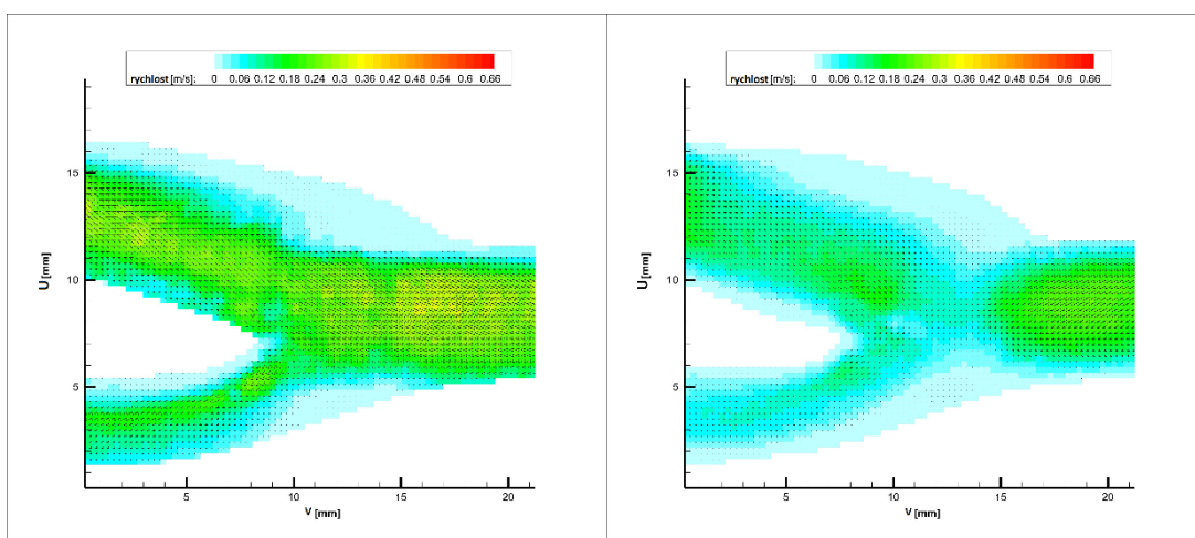
Obr. 30 Porovnání Epoxid/PDMS krevní fantom 6,267 ml/s
