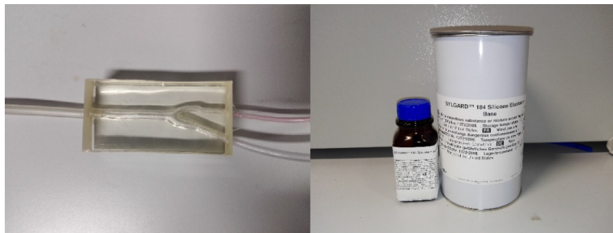
Obr. 14 a) hotový PDMS model b) dvousložkový materiál pro odlití modelu [foto autor]
