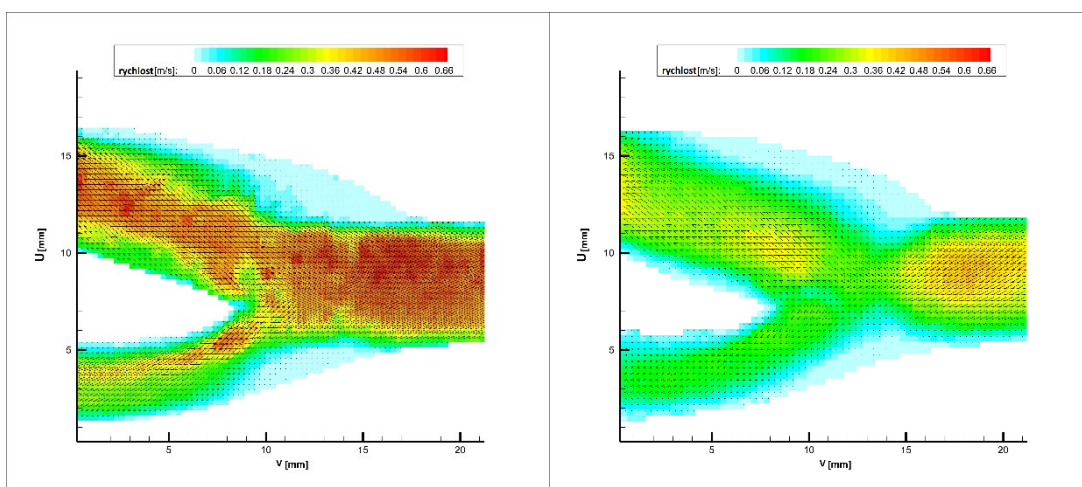
Obr. 31 Porovnání Epoxid/PDMS krevní fantom 13 ml/s
