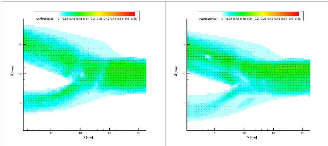
Obr. 23 Porovnání Epoxid/PDMS voda 4 ml/s
