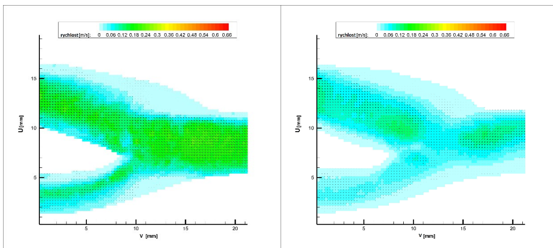
Obr. 29 Porovnání Epoxid/PDMS krevní fantom 4 ml/s
