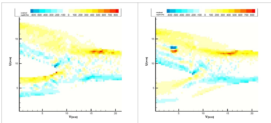
Obr. 28 Porovnání Epoxid/PDMS voda 13 ml/s
