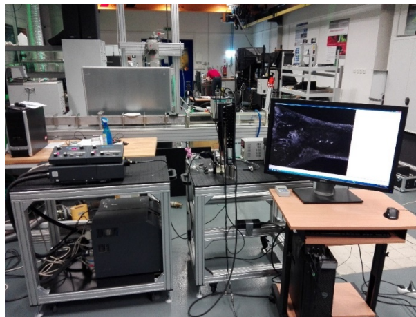
Obr. 6 Sestava experimentu [foto autor]
