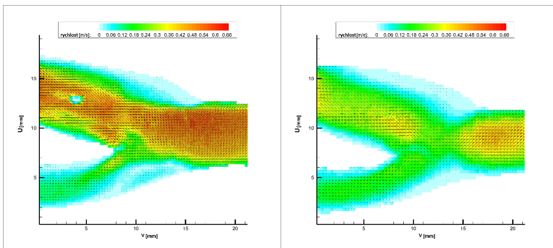
Obr. 36 Porovnání PDMS voda/krevní fantom 13 ml/s
