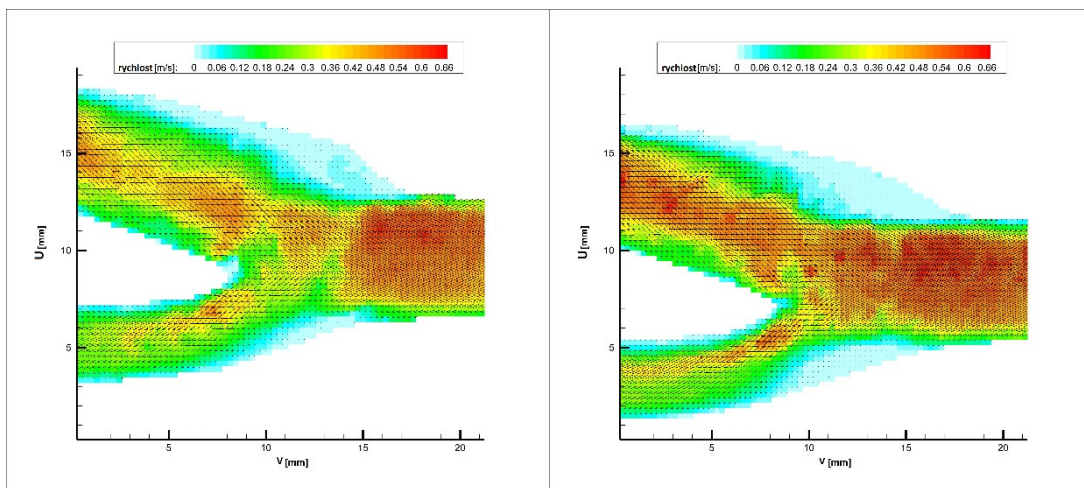
Obr. 35 Porovnání Epoxid voda/krevní fantom 13 ml/s
