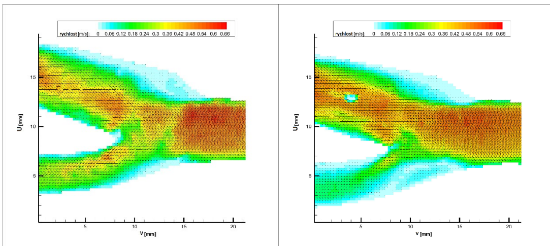
Obr. 25 Porovnání Epoxid/PDMS voda 13 ml/s
