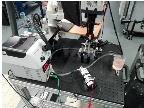
Obr. 7 Detail na experimentální trať [foto autor]
