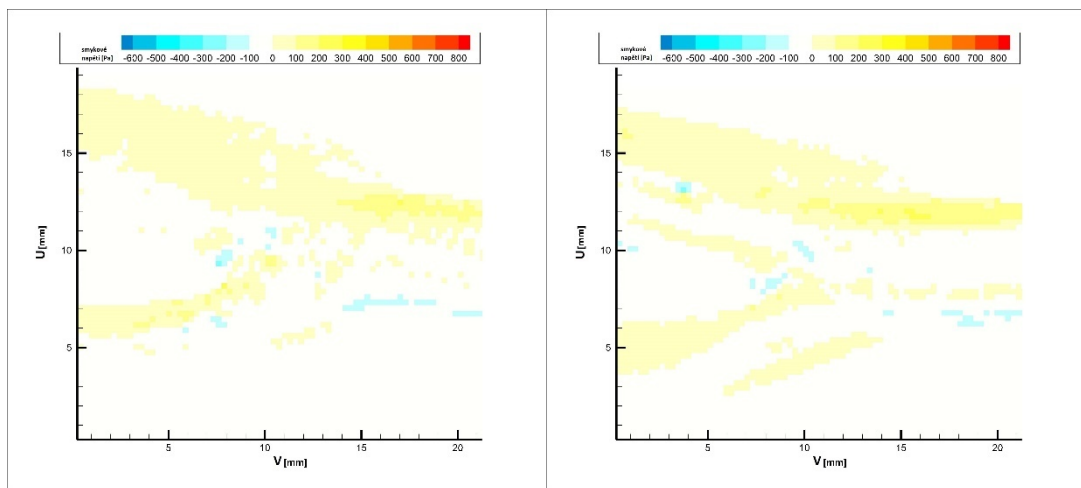
Obr. 26 Porovnání Epoxid/PDMS voda 4 ml/s
