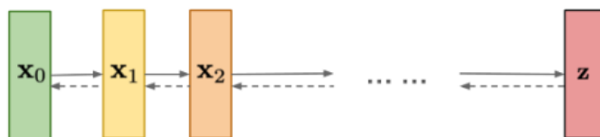
Obr. 1.9: Difuzní model postupné přidání šumu a následné odebrání při opačném postupu[9]
