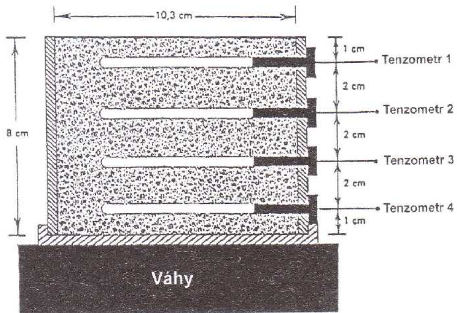
obr. č.10. Evaporační metoda
