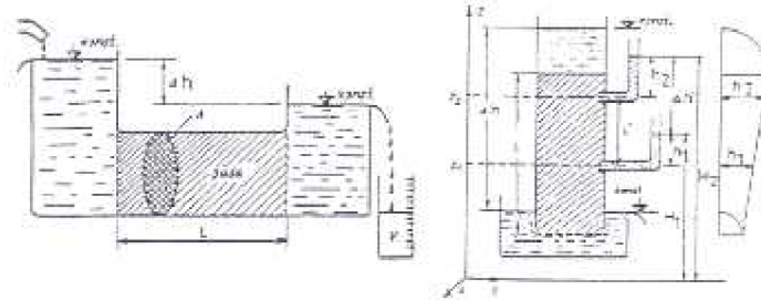
obr. č.2. Stacionární proudění sloupcem půdy o průřezové ploše A , a tlakové poměry při proudění vody sloupcem homogenní půdy (převzato: Kutílek a kol., 1993)
