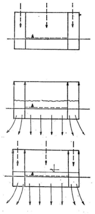
obr. č.17. Způsob provedení infiltračního pokusu (převzato časopis Vodní hospodářství č. 5, 1988)
