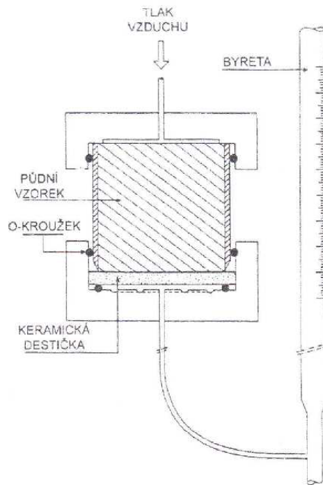
obr. č.9. Tempská cela
