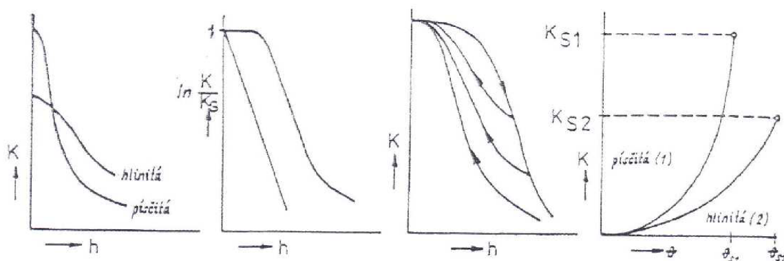
obr. č.7. Závislost nenasycené vodivosti K na záporné tlakové výšce a na vlhkosti \theta (převzato Kutílek a spol. 2000)
