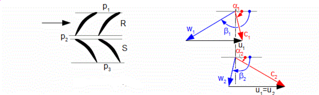
Obrázek 8 - rychlostní trojúhelník [10]
