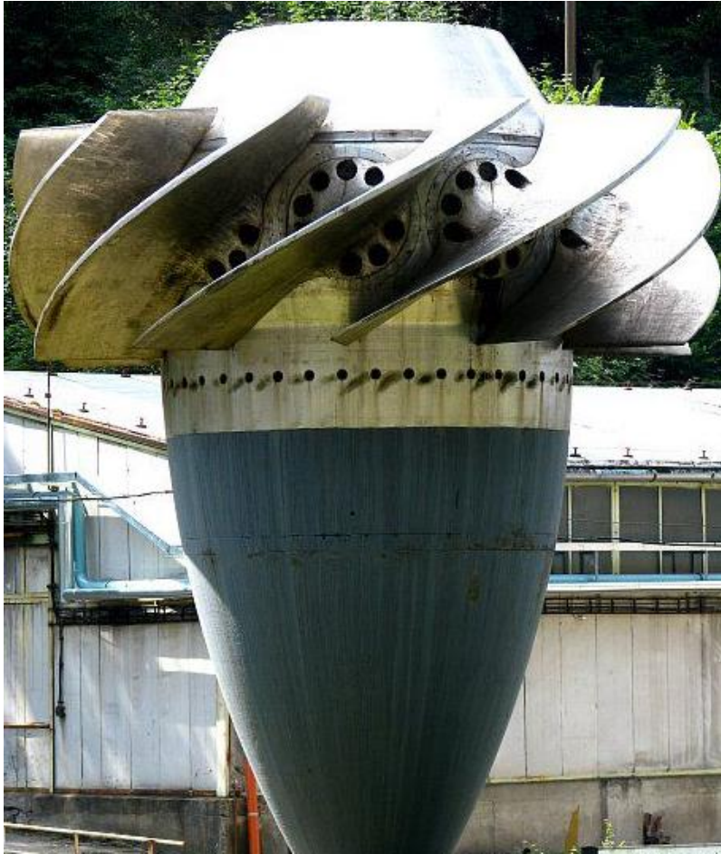
Obrázek 2 - Kaplanova turbína [2]
