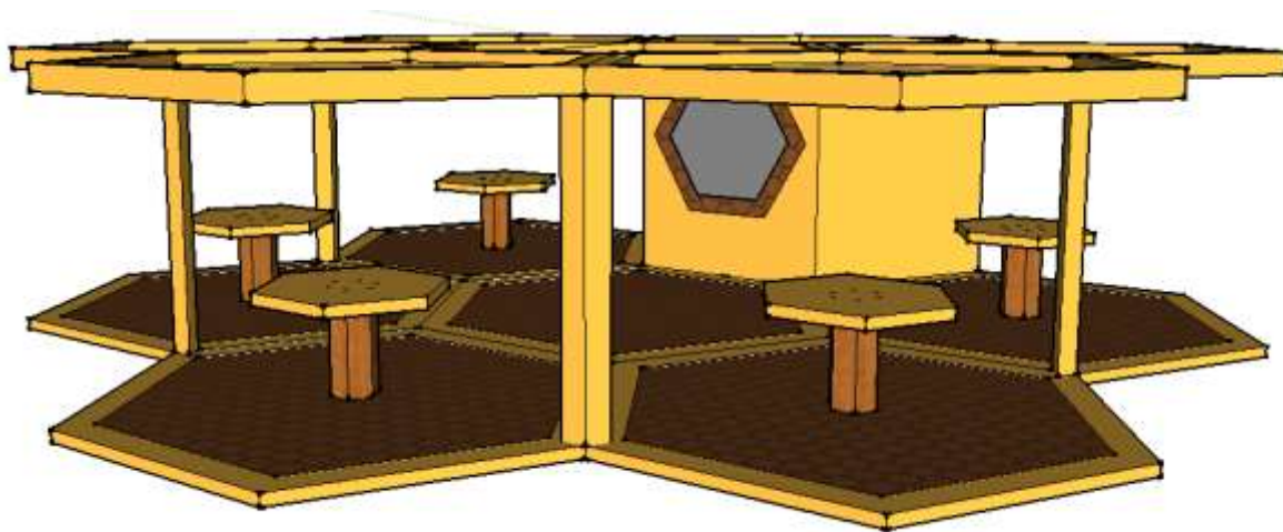
Obr. č. 36 - Boční pohled na kiosek; vlastní návrh autora
