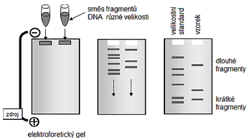
Obrázek 3: Gelová elektroforéza [5]
