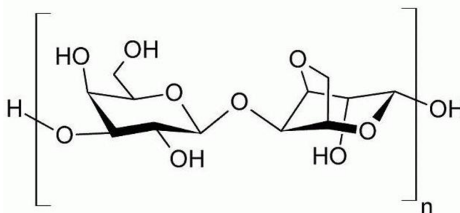
Obrázek 1: Struktura agarózy [1]
