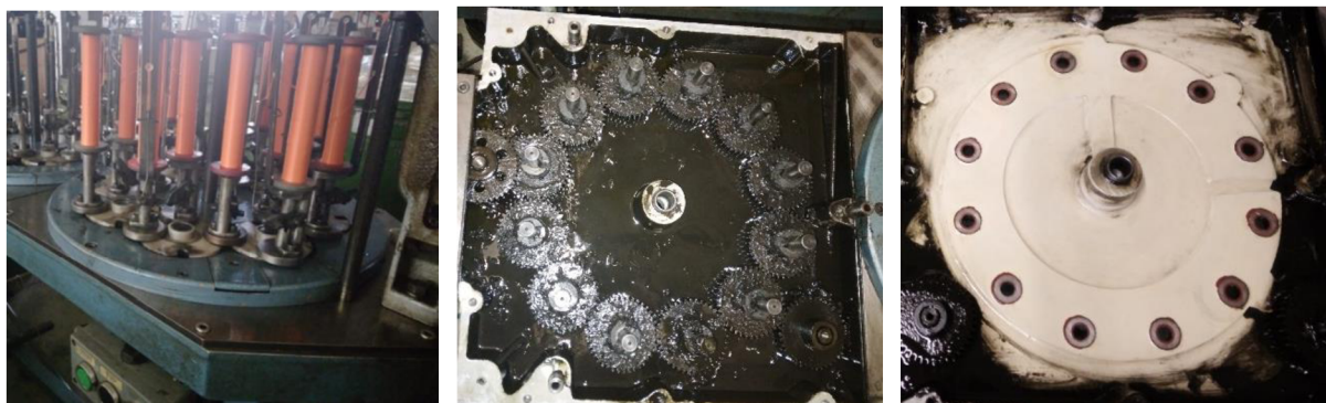
a) b) c) Obrázek 9. Olejová vana vlevo se soukolím a)zvenku, b)uvnitř, c)bez soukolí
