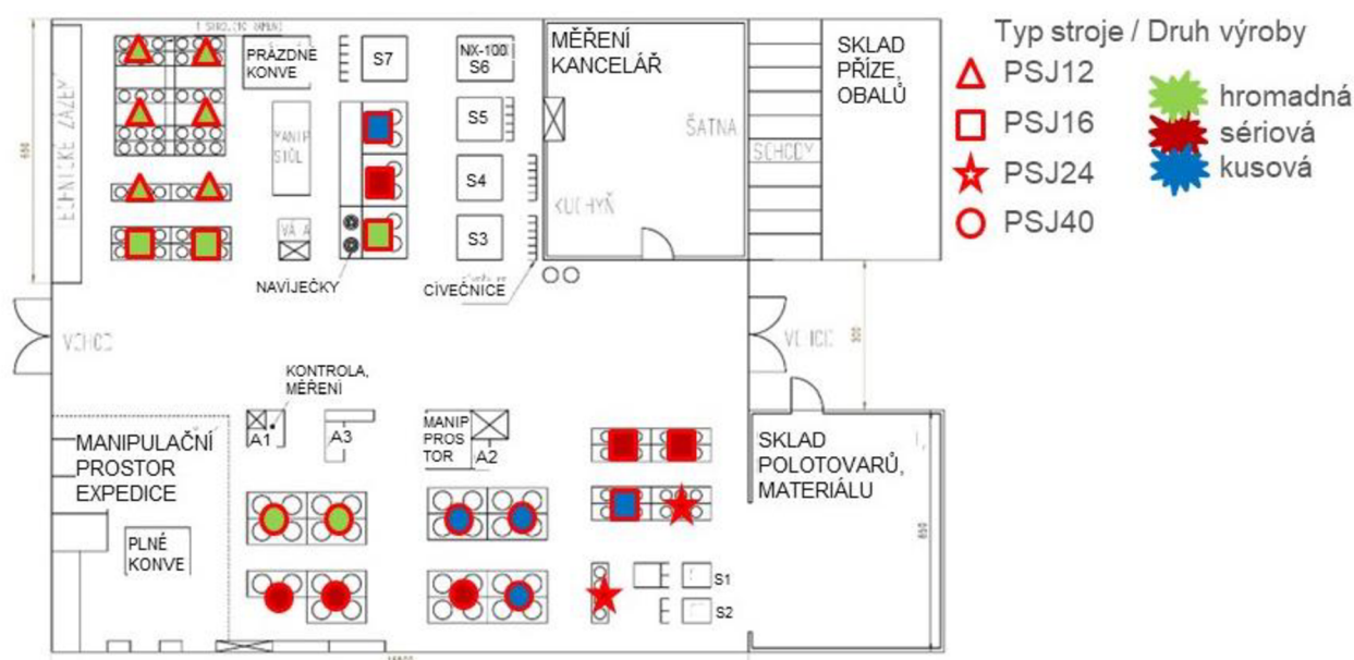
Obrázek 30. Nový layout pletárna
