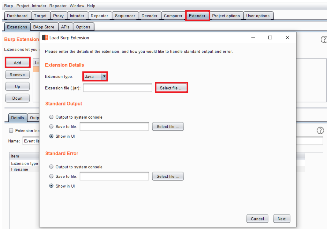
Obr. 2.4: Pridanie modulu.
