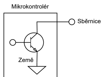
Obrázek 2.2: Open drain
