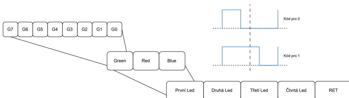
Obrázek 2.9: Komunikační protokol pro WS2812 led
