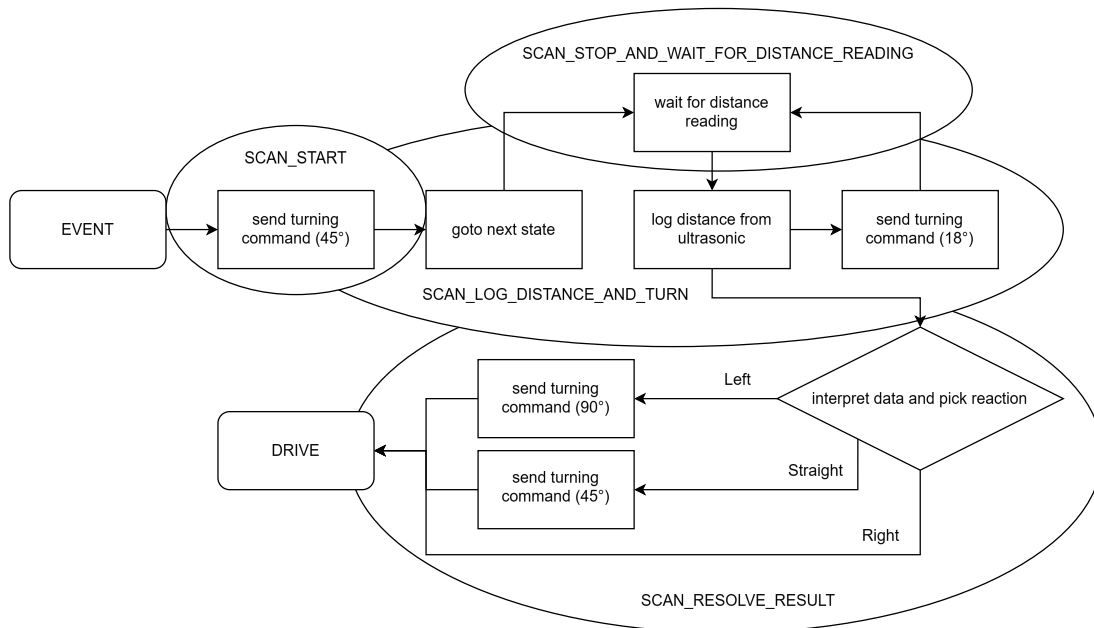
Obrázek 4.13: Algoritmus preventivního hledání překážek.
