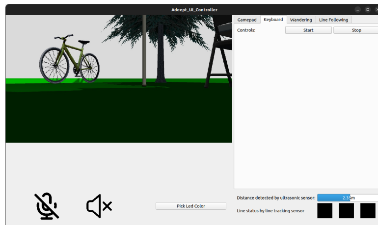
Obrázek 4.15: Uživatelské rozhraní
