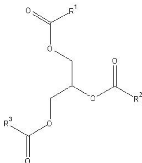
Obrázek 2.2: Triacylglycerol
