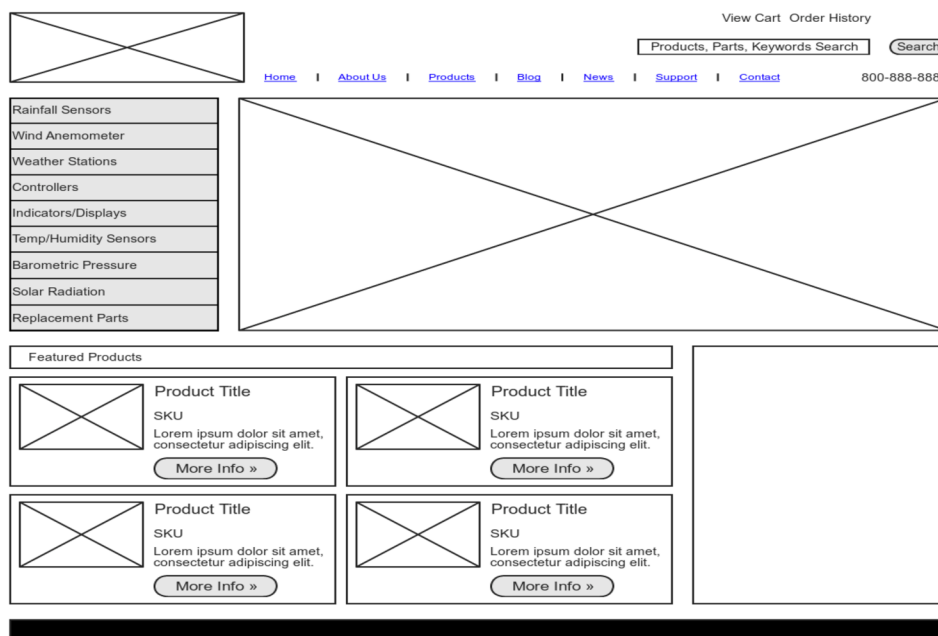
Obrázek 9: Wireframe [9]
