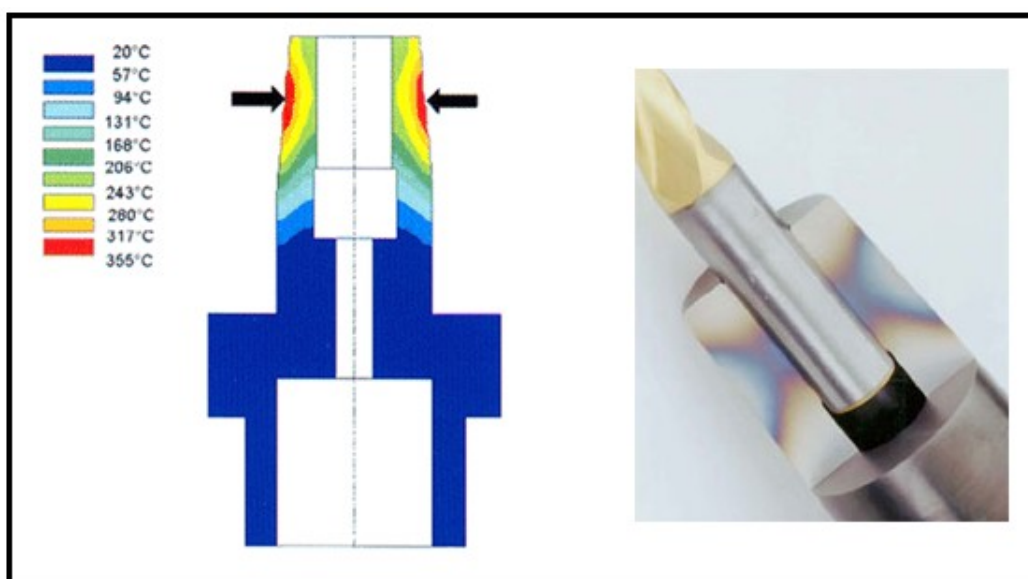
Obr. 3.4 Řez tepelným upínačem typu ThermoGrip s upnutým nástrojem. [24]
