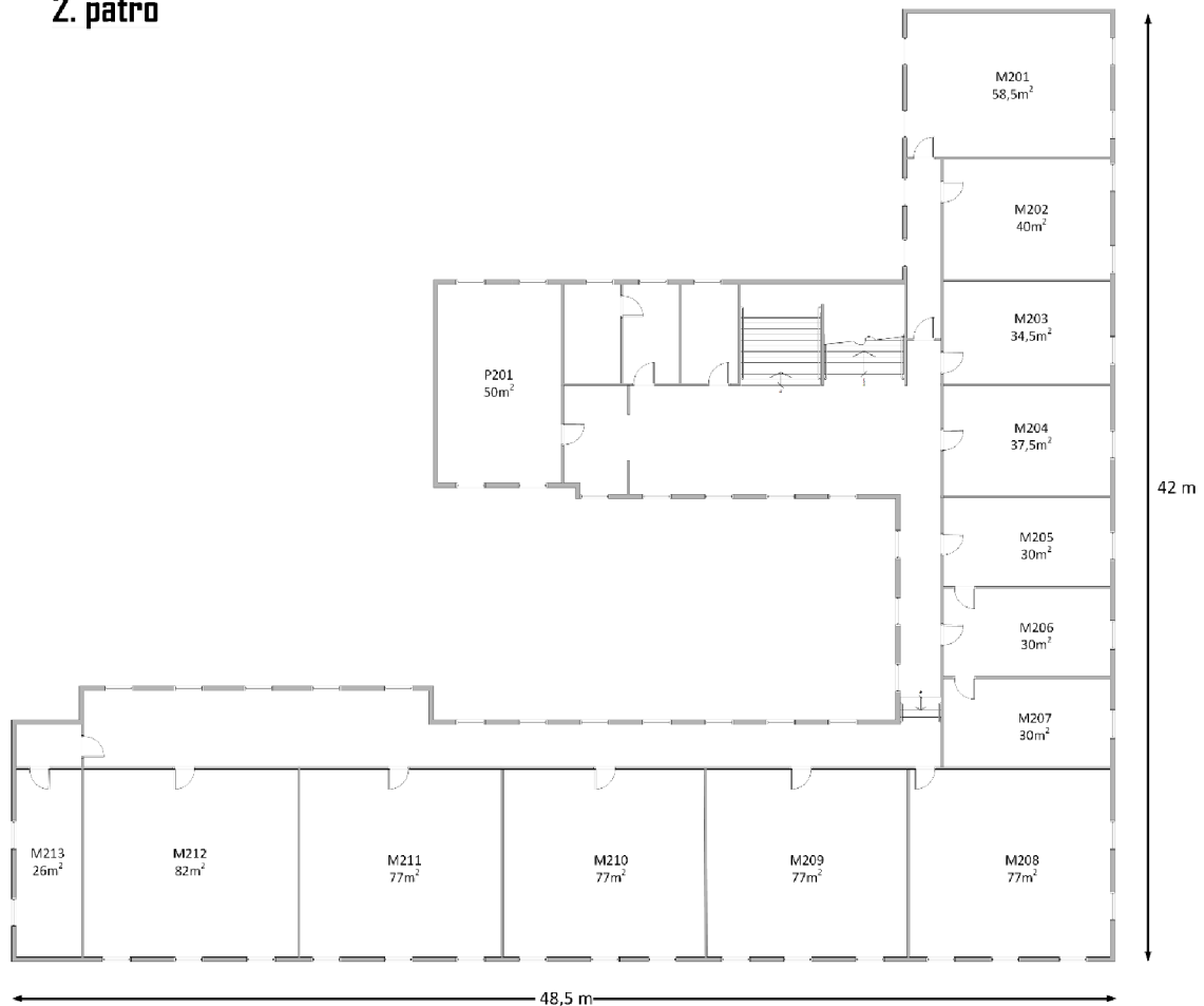
Obrázek 2: Půdorys 2.NP
