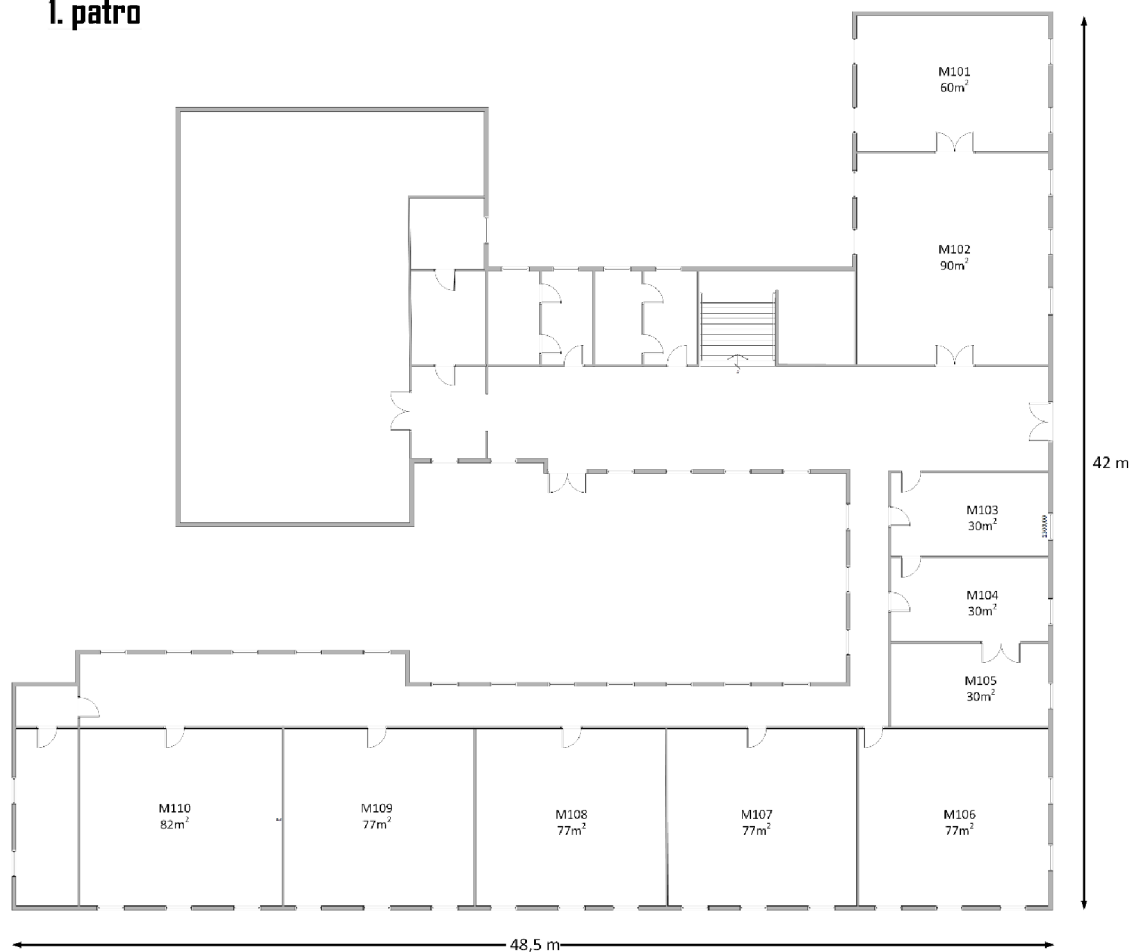
Obrázek 1: Půdorys 1.NP
