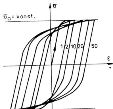
Obr. 4.9 Hysterezní smyčka [8]
