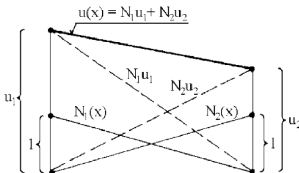
Obr. 4.24 Báзовé funkce prutového prvku [11]
