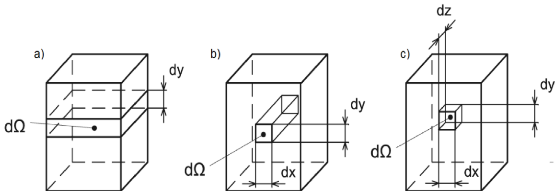
Obr. 4.2 Elementární prvky [5]
