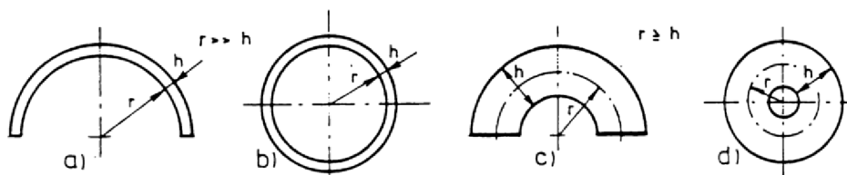
Obr. 4.17 Zakřivené pruty [6]
