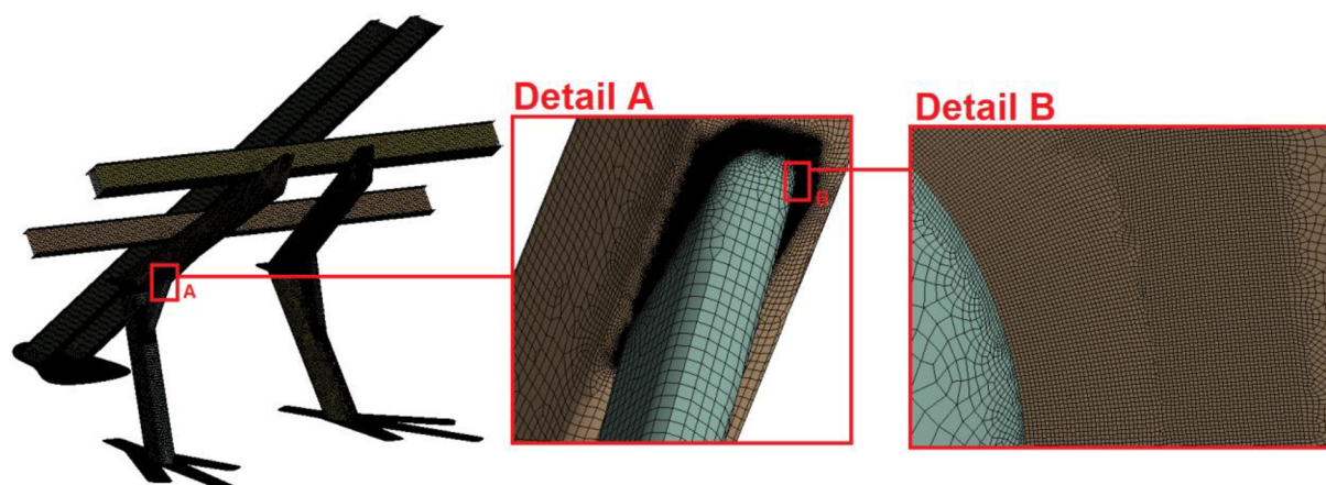
Obr. 5.5 Konečnoprvková síť [13]
