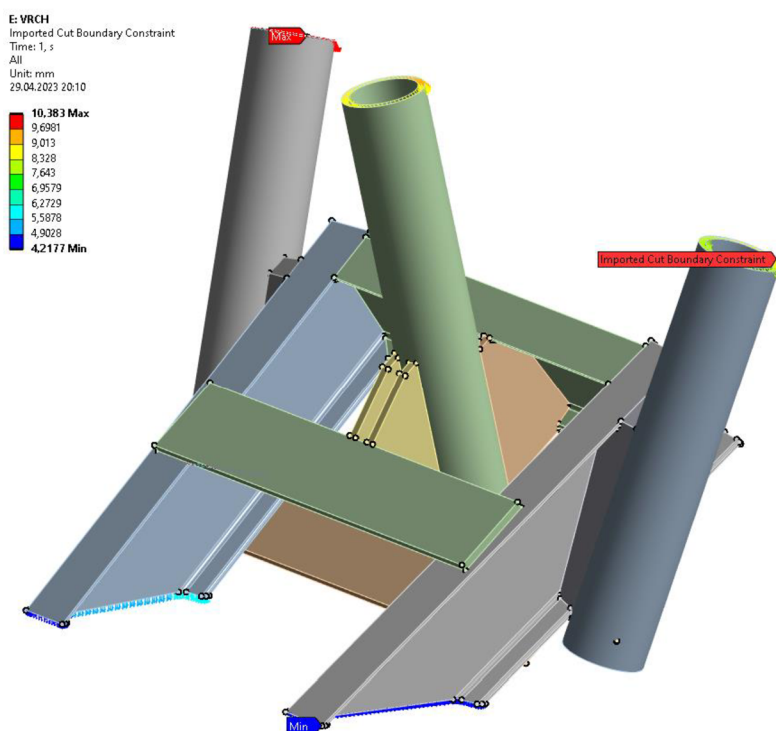
Obr. 7.13 Importované deformace na submodelu uchycení krků
