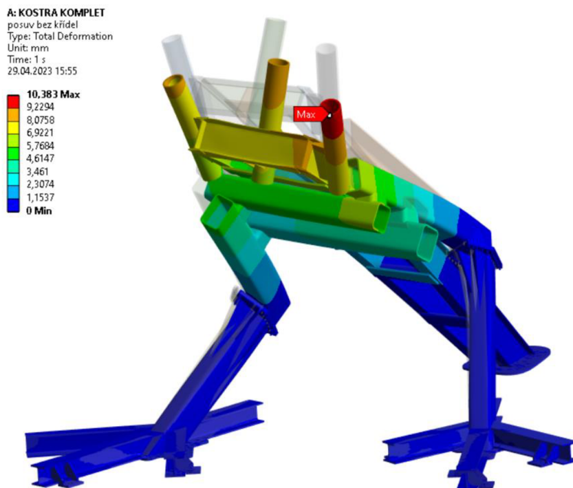
Obr. 7.7 Celkové deformace konstrukce bez křidel
