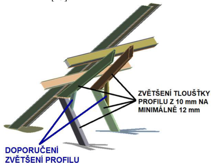
Obr. 5.7 Znáornění navržených úprav [13]
