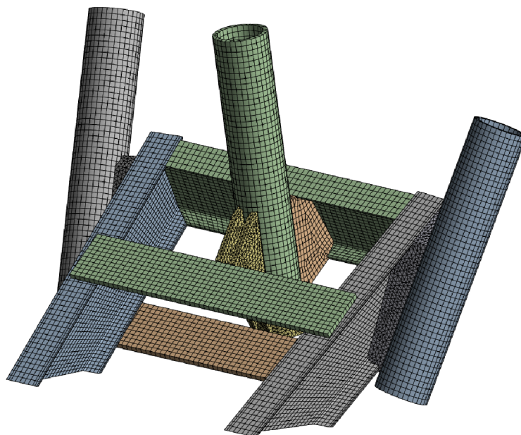
Obr. 7.12 Tvar sítě submodelu uchycení krků
