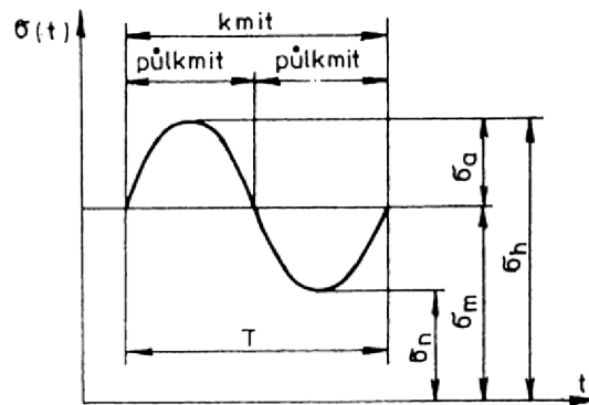
Obr. 4.7 Průběh harmonického napětí [8]
