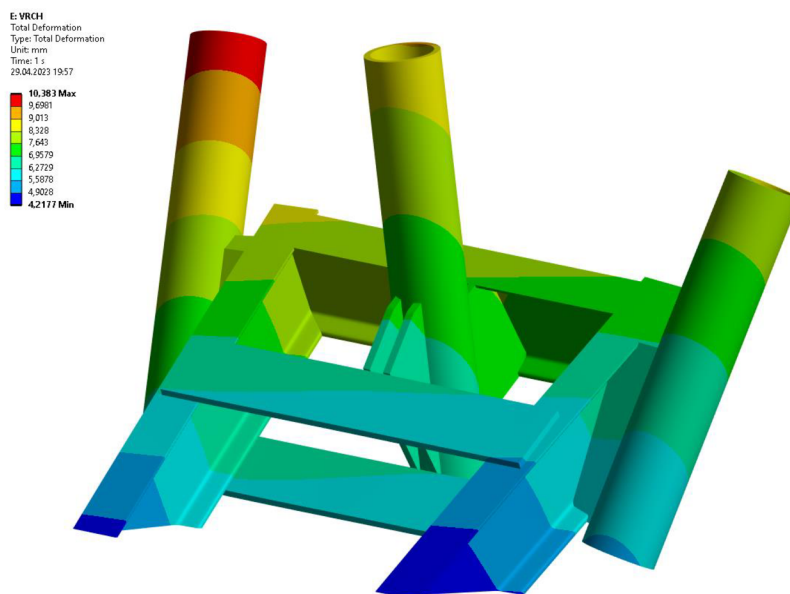
Obr. 7.14 Deformace submodelu uchycení krkú
