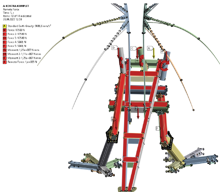
Obr. 7.5 Zatížení konstrukce
