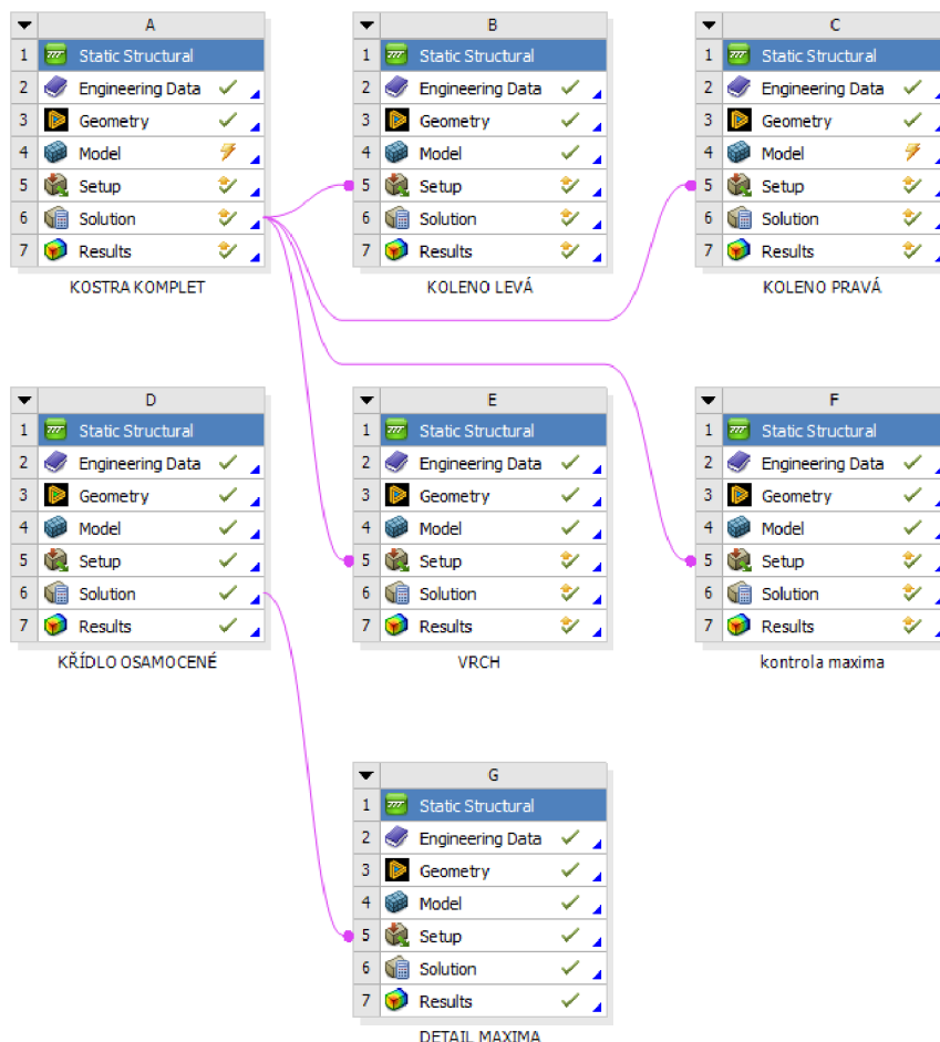
Obr. 7.2 Použité analýzy
