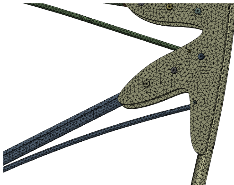
Obr. 7.24 Detail síť křídla
