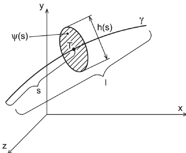
Obr. 4.10 Geometrické předpoklady [5]
