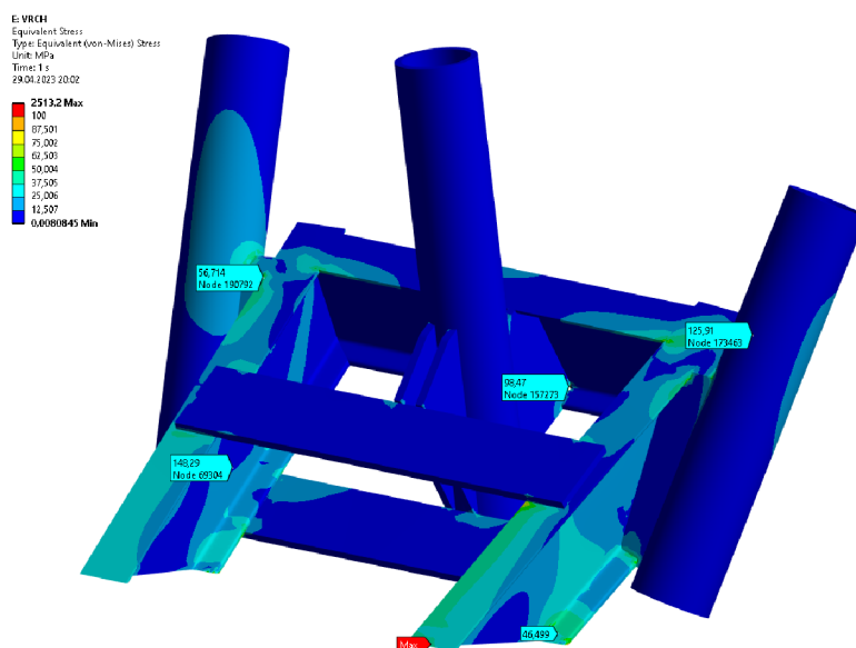
Obr. 7.15 Redukované napětí na submodelu uchycení krkú
