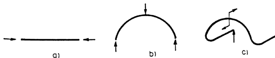
Obr. 4.14 Geometrie prutu [6]
