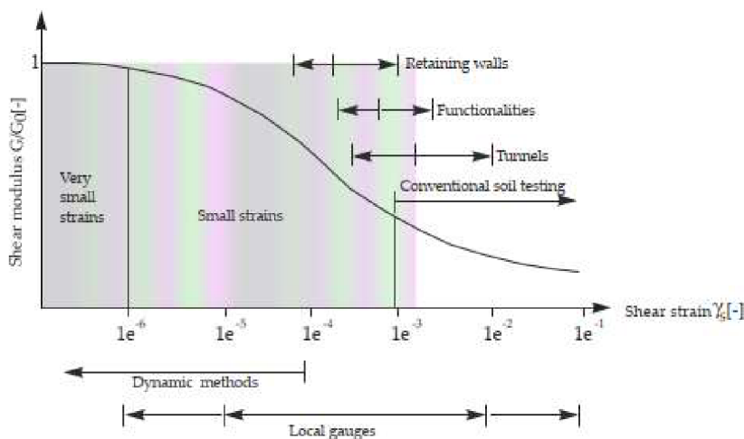
Obr. 3.9 Tuhostně-deformační chování zemin s běžnými rozsahy deformace pro laboratorní zkoušky a konstrukce [13].
