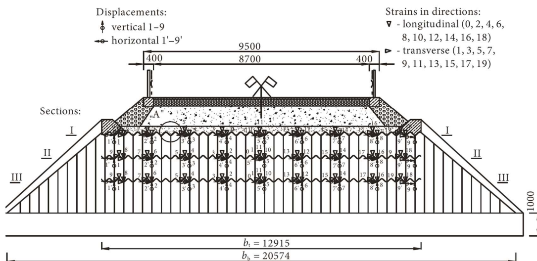
Obr. 2.10 Příčný řez – měřící body posunů 1-9 a 1'-9' číslovány zleva doprava (schéma platné pro měření při hutnění i zatěžovém testu), měřící body přetvoření 0 – 9 číslovány od osy doleva a měřící body přetvoření 10 – 19 číslovány od osy doprava (schéma platné pro měření při hutnění) [2].
