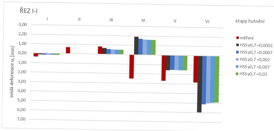
Graf 4-3 Porovnání vodorovných deformací v jednotlivých řezech pro modely s HSS
