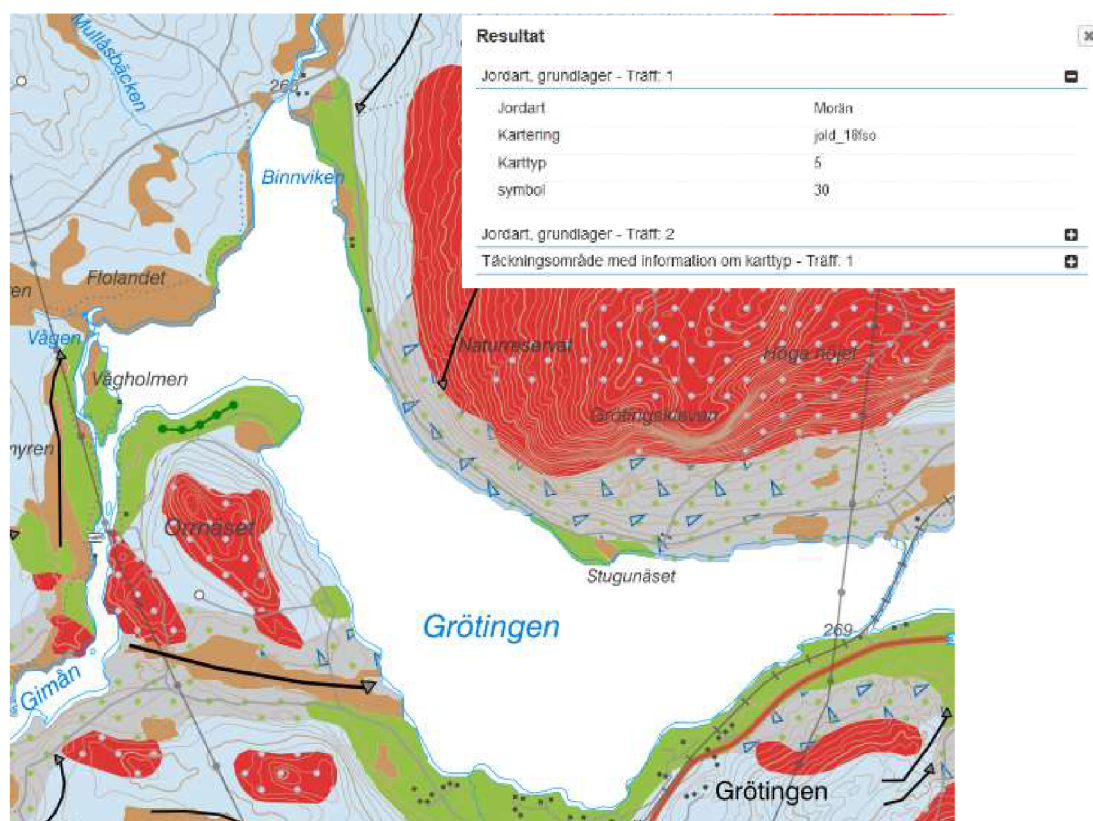
Obr. 2.5 Kvarterní vrstvy [9].
