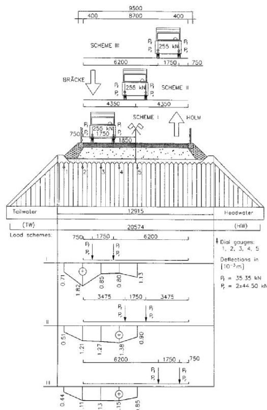
Obr. 2.14 Grafy maximálních vertikálních posunů pro jednotlivá schémata zatěžovací zkoušky [3].
