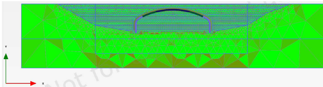
Obr. 3.11 Vygenerovaná síť konečných prvků – typický 2D model
