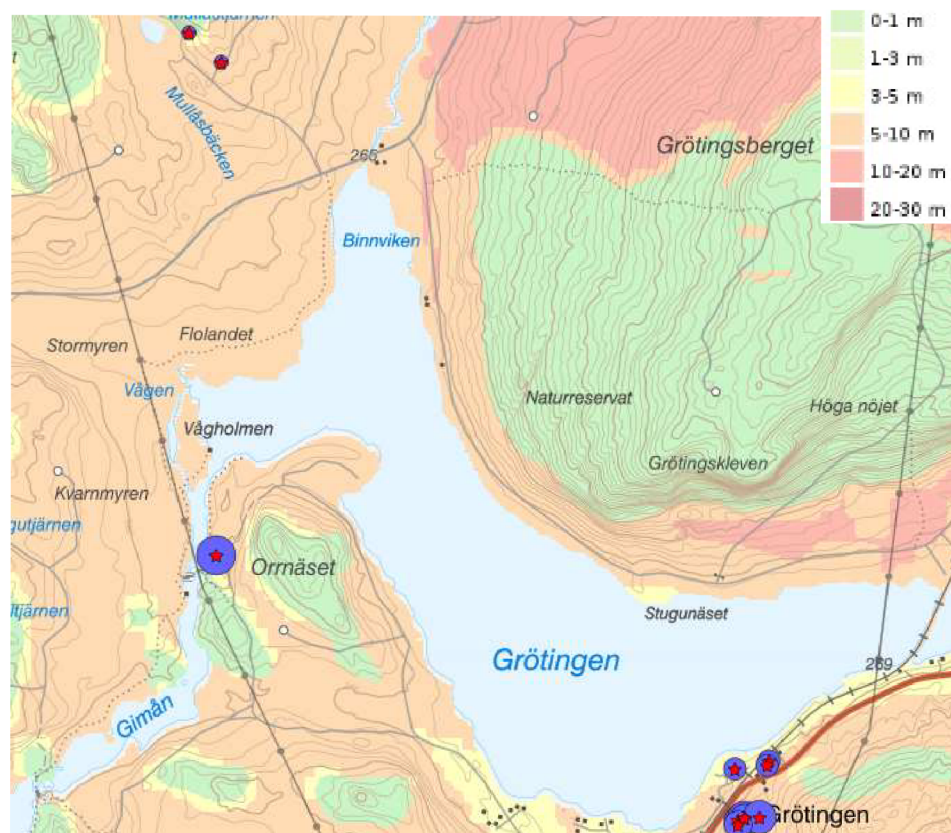
Obr. 2.4 Mocnost kvartéru [8].
