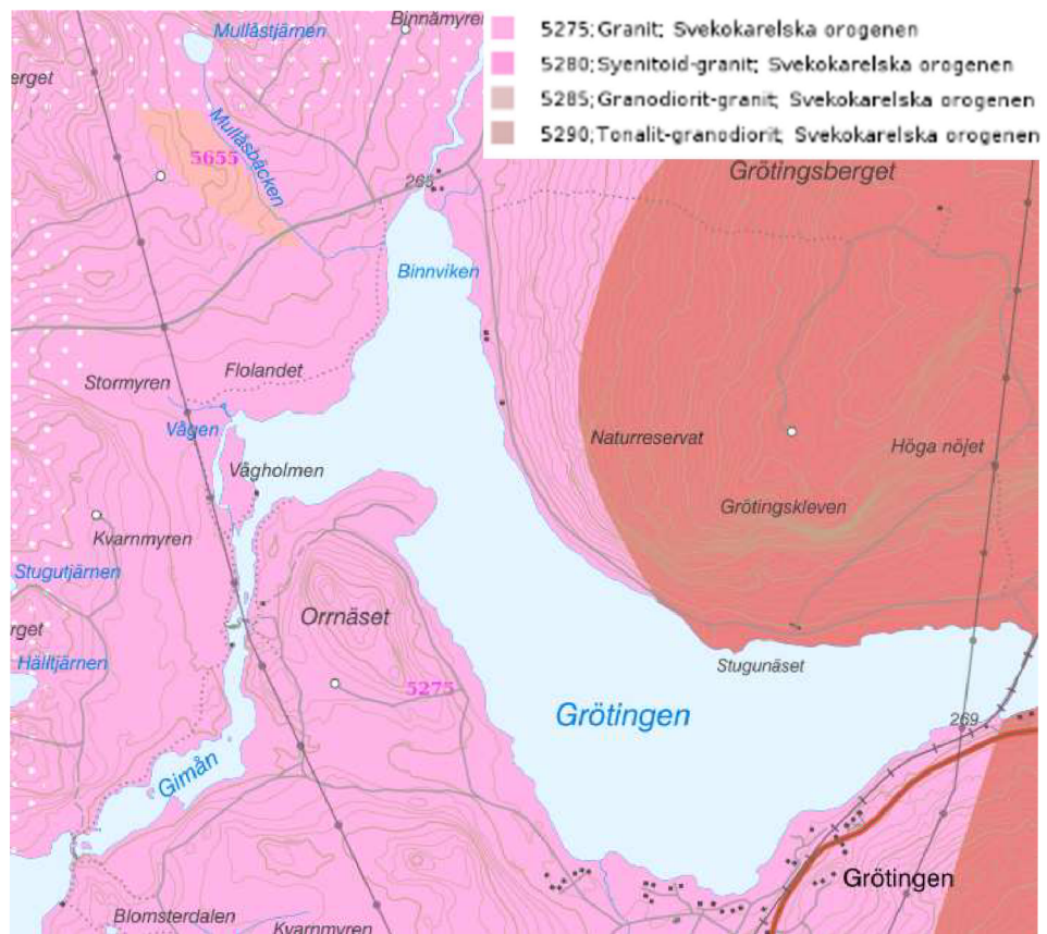
Obr. 2.3 Předkvartérní podloží [7].
