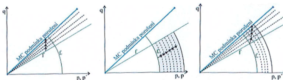
Obr. 3.7 Znárodnění ploch plasticity v rovině p-q, vlevo – smykové zpevnění, uprostřed – objemové zpevnění, vpravo – kombinované zpevnění zeminy [12].
