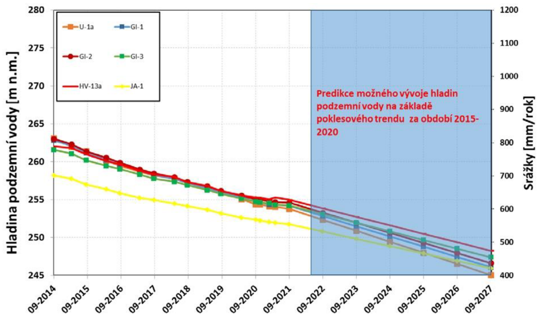
Obr. 10: Předpokládaný vývoj stavu hladin v kvartérním a svrchním terciérním kolektoru v okolí Uhelné (převzato z: Venera a kol., 2021).
