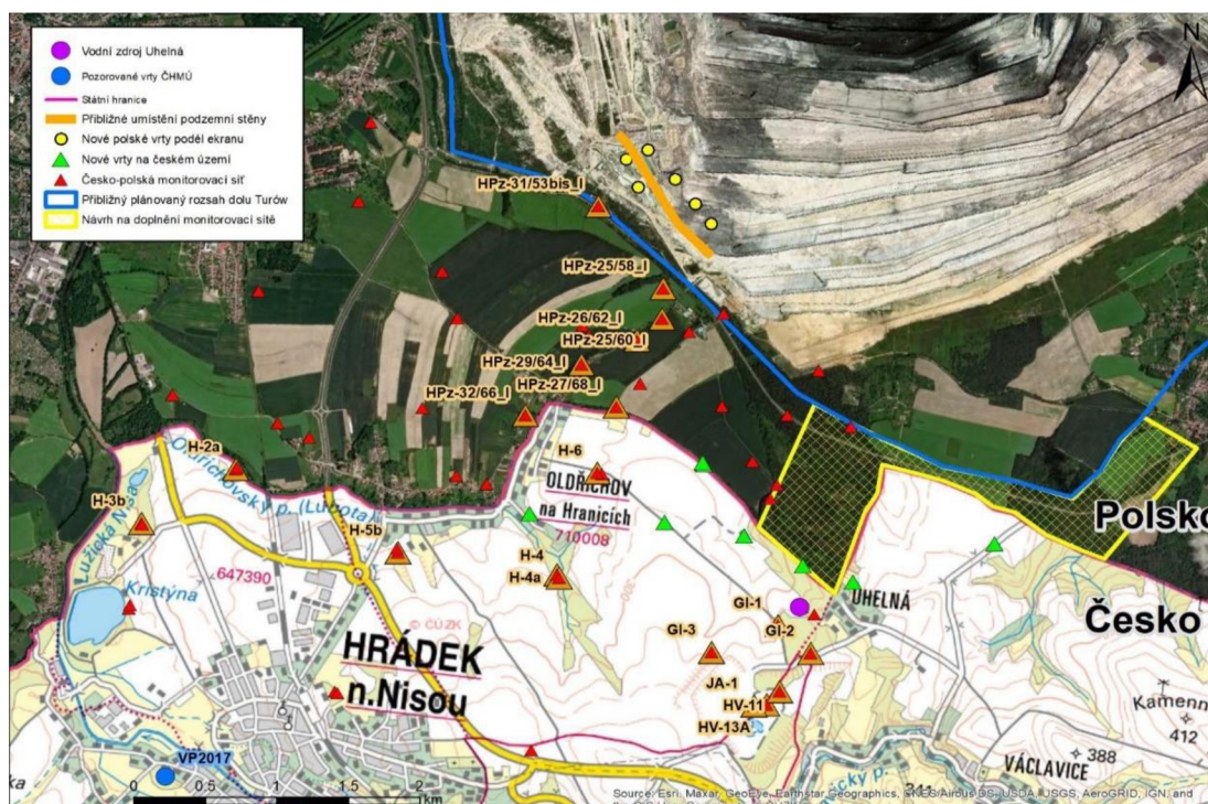
Obr. 5: Monitorovací vrty v hrádecké části Žitavské pánve (převzato z: Venera a kol., 2021).
