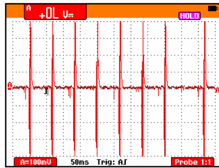
Obr. 4.7 Průběh napěťového signálu na plošce (vzorek č. 5)
