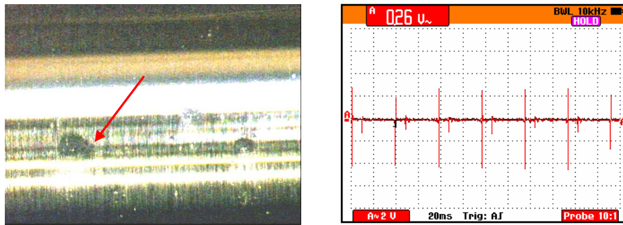
Obr. 4.11 Průběh napětového signálu na vtisku (vzorek č. 9)
