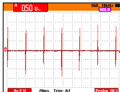
Obr. 4.10 Průběh napěťového signálu na lunkru (vzorek č. 8)
