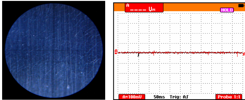
Obr. 4.4 Signál získaný na povrchu pístitnice bez vady
