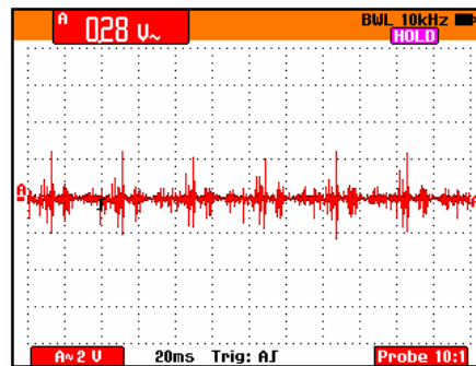
Obr. 4.9 Průběh napěťového signálu na nedobroušeném povrchu (vzorek č. 2)
