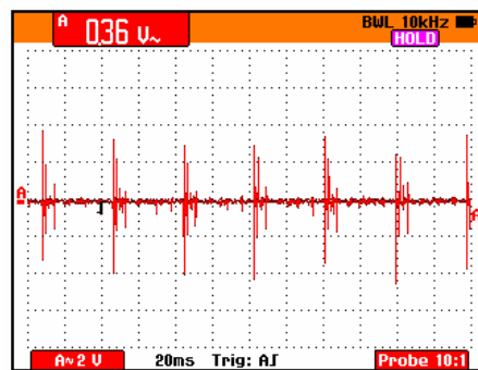
Obr. 4.8 Průběh napěťového signálu na záseku (vzorek č. 3)
