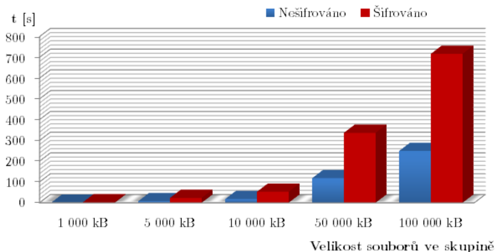
Obr. 3.14: Graf závislosti velikosti souborů na čase kopírování - druhá část
