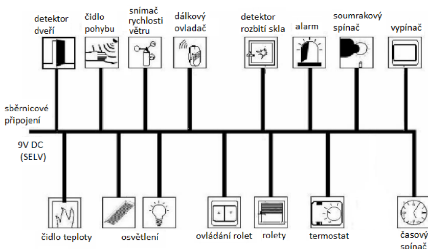
Obrázek 2-2-2 Příklad sběrnicevých elektroinstalace [24]
