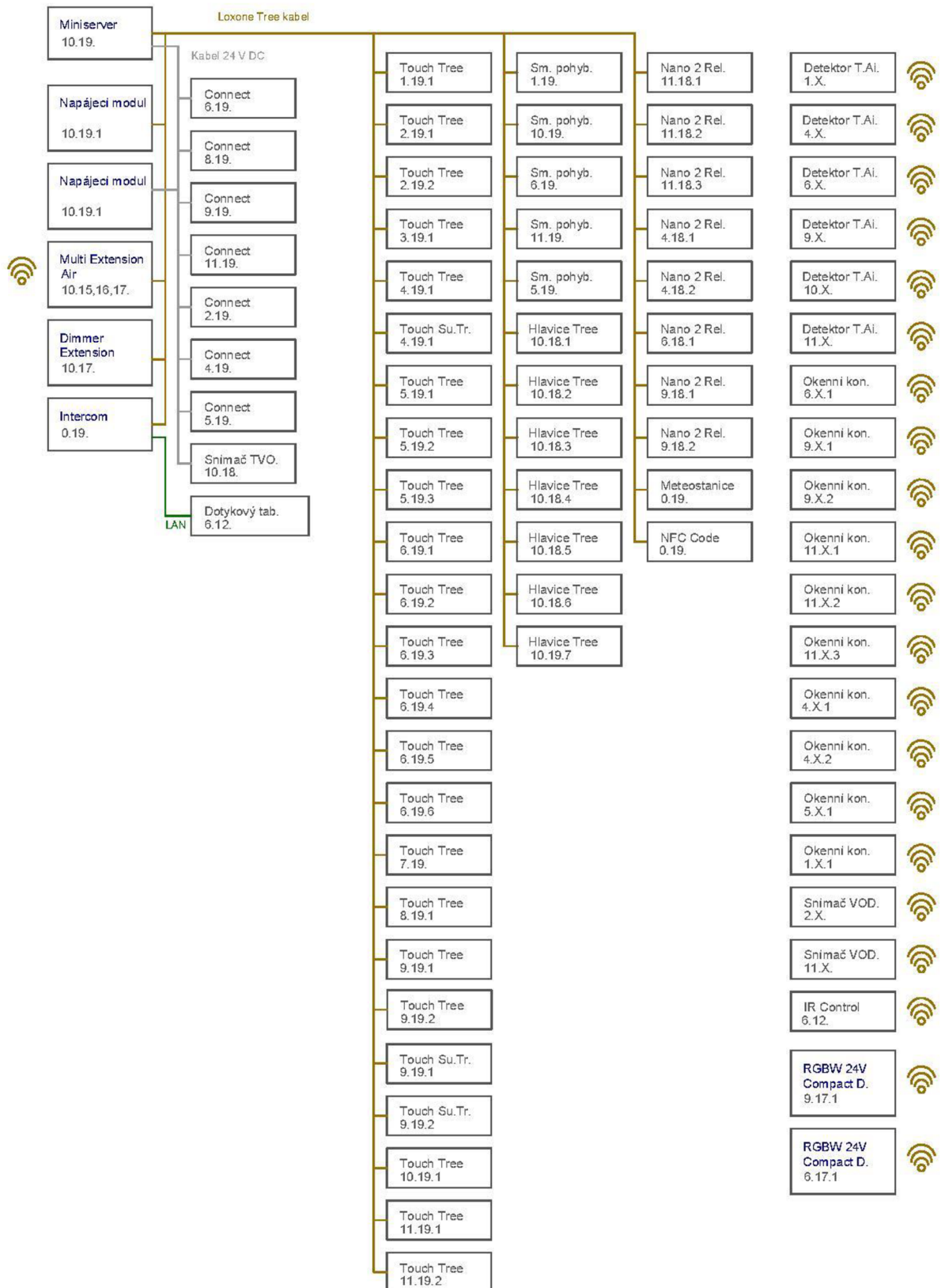
Obrázek 4-2 Blokové schéma Loxone
