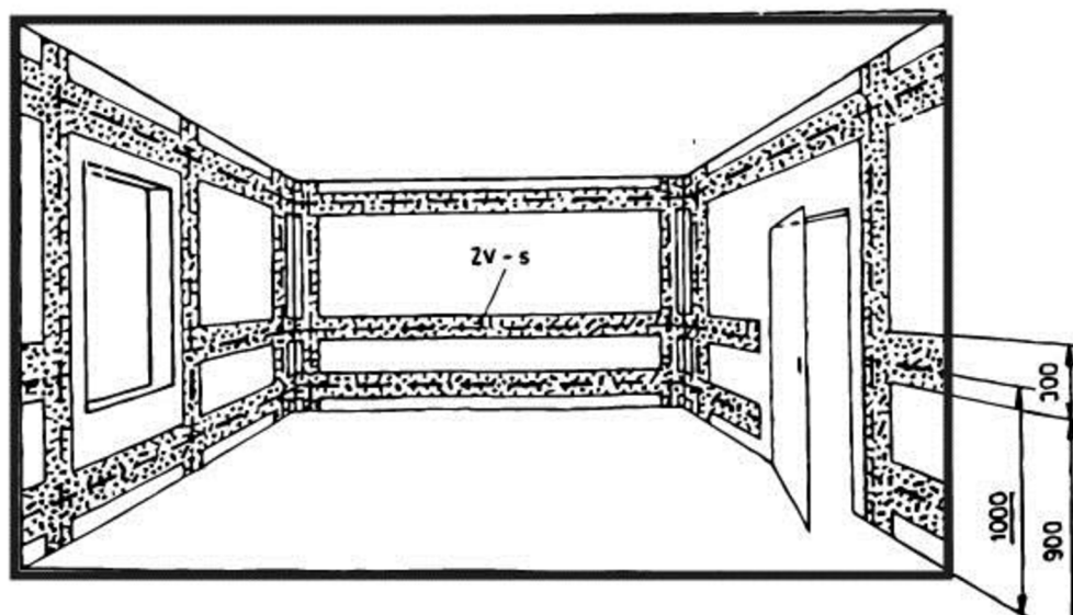
Obrázek 5-2 Instalační zóny 2 [6]
