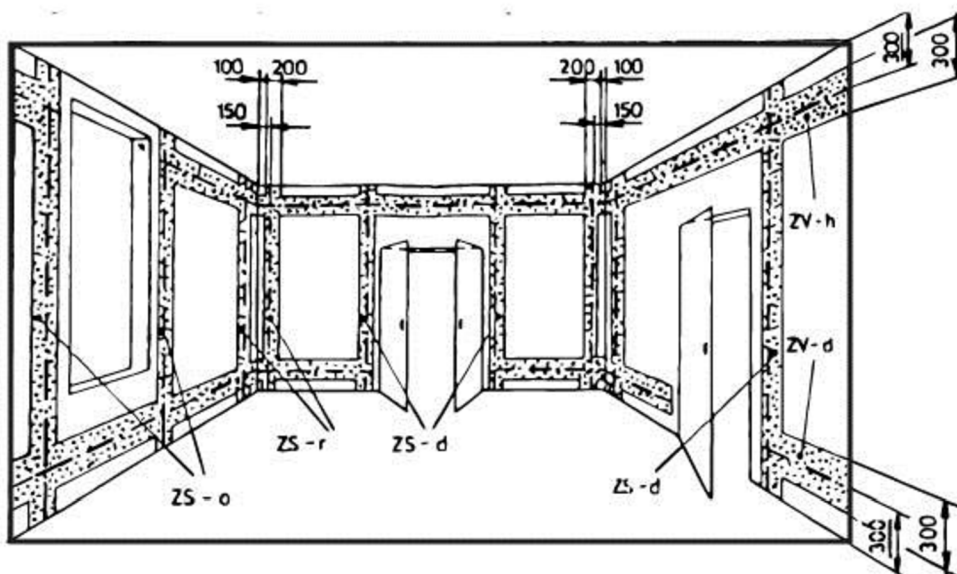
Obrázek 5-1 Instalační zóny 1 [6]
