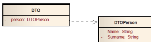
Obrázek č. 6: Ukázka jednoduchého DTO modelu (Zdroj: Vlastní zpracování dle: 19)
