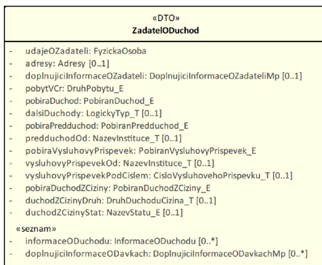
Obrázek č. 16: DTO ZadatelODuchod
