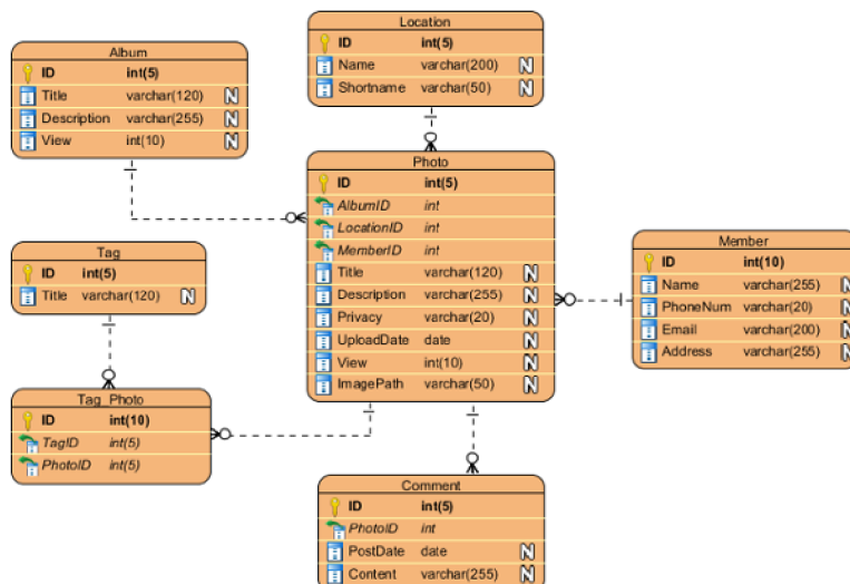
Obrázek č. 5: Ukázka fyzického uložení tabulek v databázi (Zdroj: 17)
