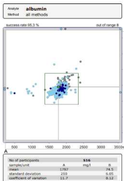
Obrázek 8 Grafické vyhodnocení výsledku EHK (Youdenův graf) Pozn.:D = rozdíl vlastní naměřené hodnoty od cílové hodnoty koncentrace albuminu, Dmax = maximální povolená diference
