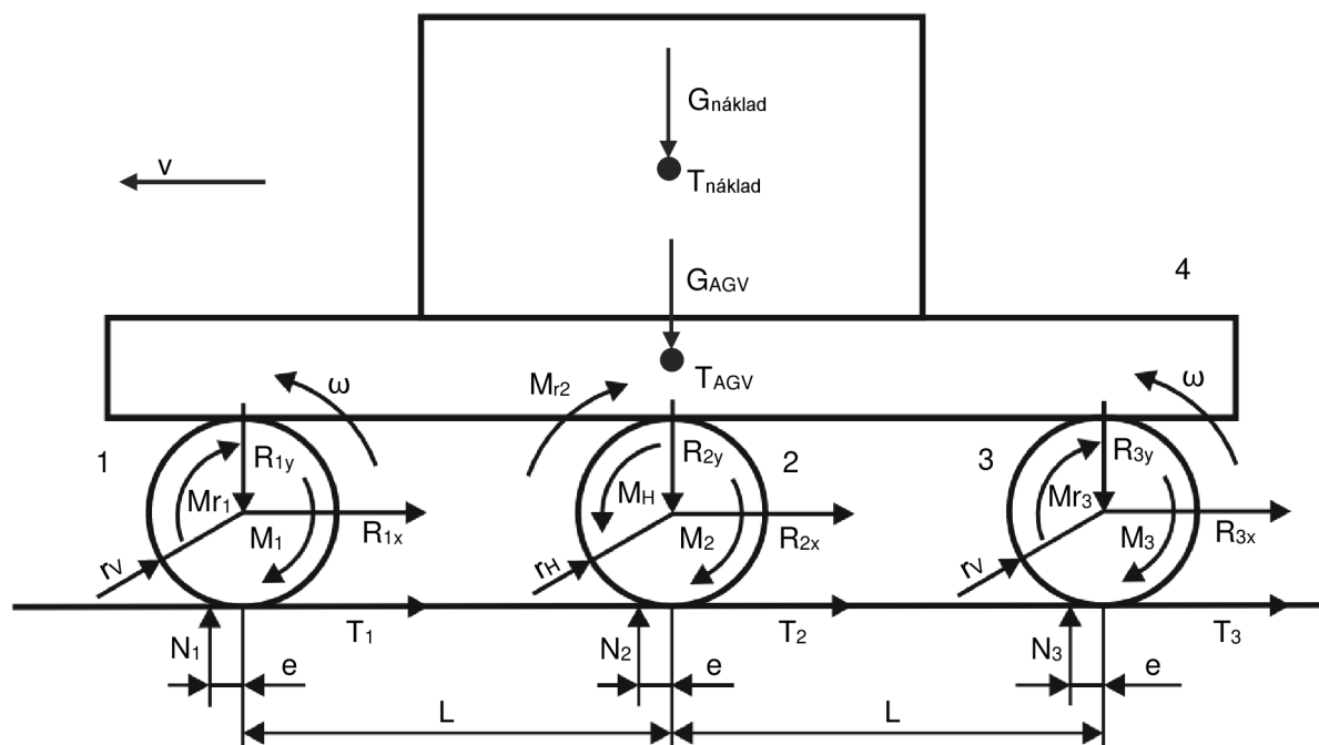
Obr. 41 Vozík – síly
