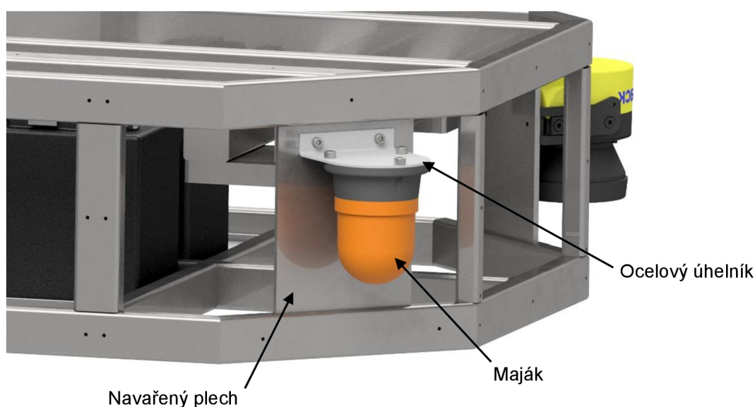
Obr. 57 Uchycení majáku
