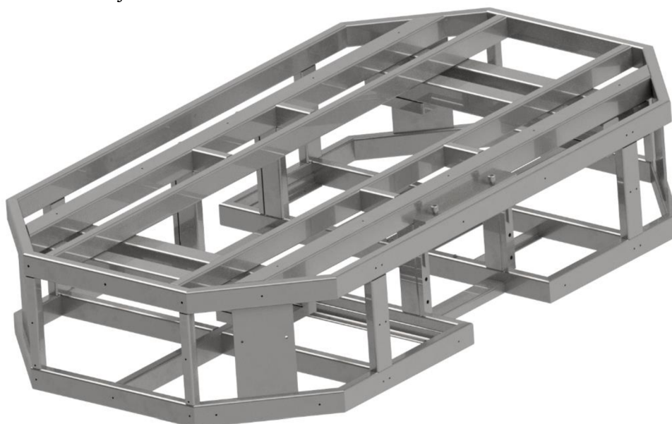
Obr. 50 Rám vozíku
