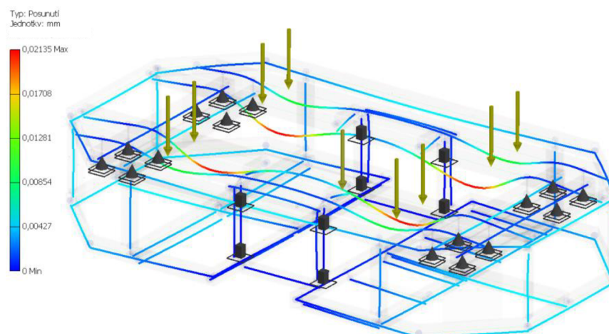
Obr. 62 Hodnoty posunutí
