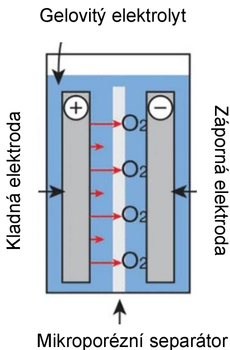
Obr. 15 GEL akumulátor [44]
