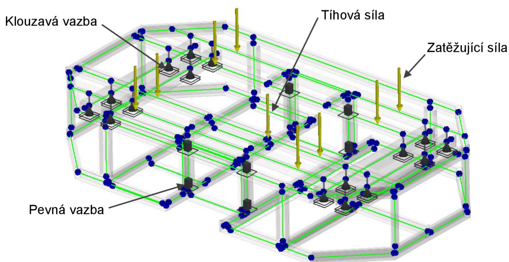
Obr. 61 Výpočtový model
