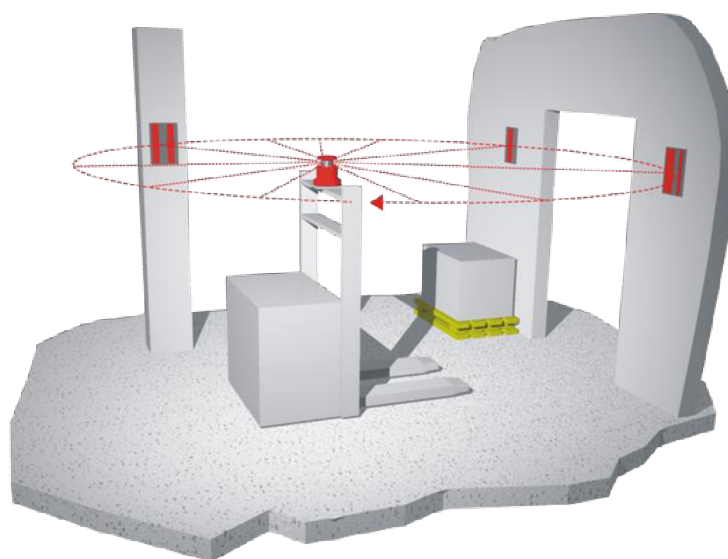
Obr. 28 Laserová navigace [10]
