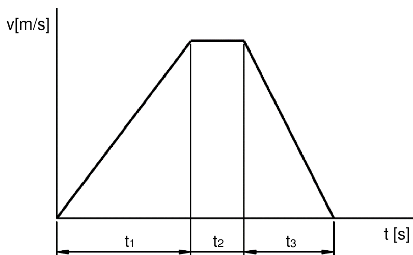
Obr. 47 Časový průběh
