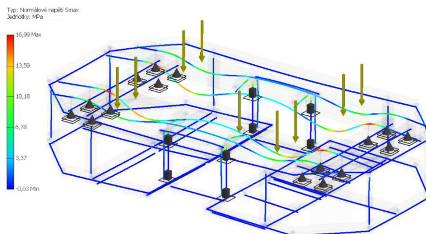
Obr. 63 Hodnoty napětí
