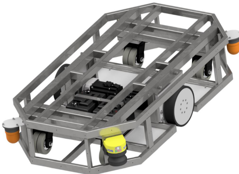
Obr. 59 Osazený rám
