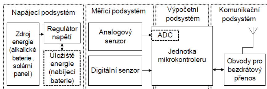
Obr.2: Schéma bezdrátového senzorového uzlu [1].
