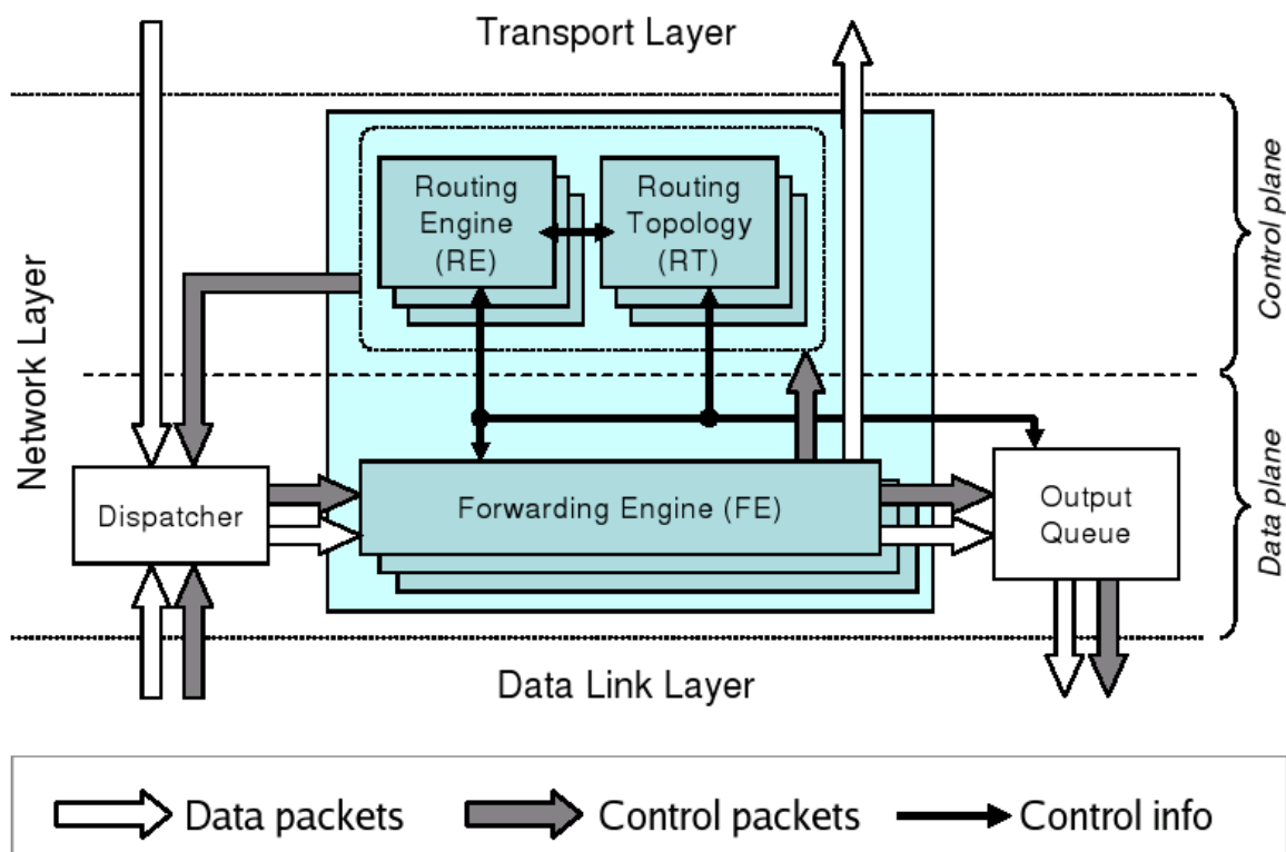
Obr.12: Síťový model představující spojení jednotlivých vrstev [6].
