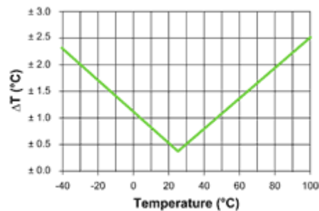
Obr.9: Přesnost měření teploty [14].
