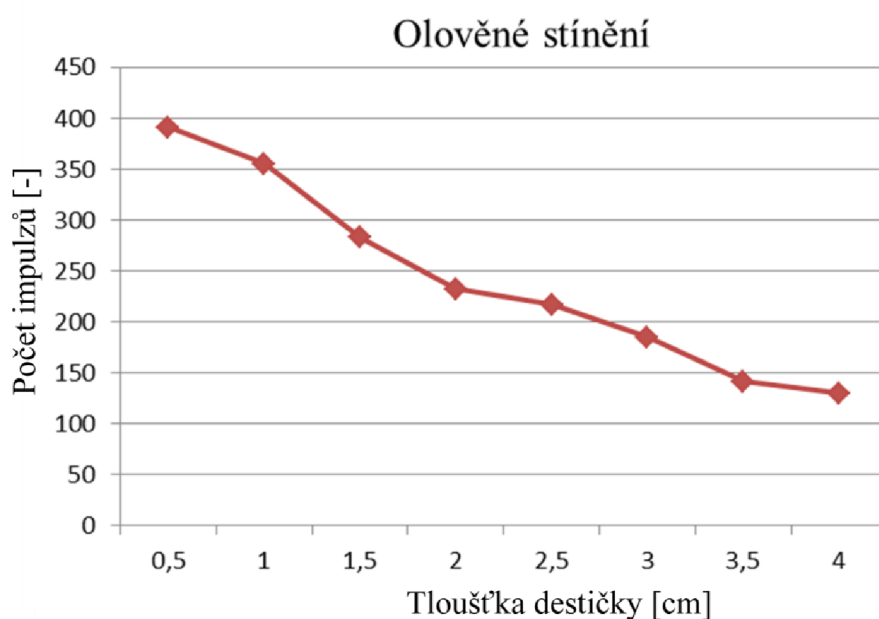
Obrázek 15: Grafická závislost počtu impulzů na tloušťce olověné destičky
