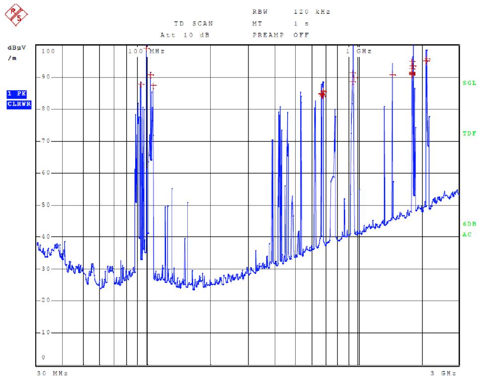
Obrázek 23: Měření vertikálně polarizované antény
