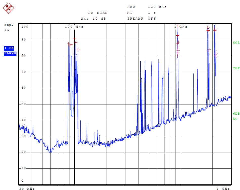
Obrázek 24: Měření horizontálně polarizované antény
