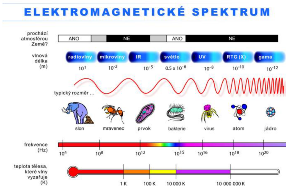
Obrázek 5: Elektromagnetické spektrum [11]
