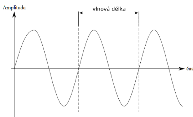
Obrázek 4: Znázornění vlnové délky [42]
