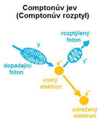
Obrázek 2: Comptonův jev [70]
