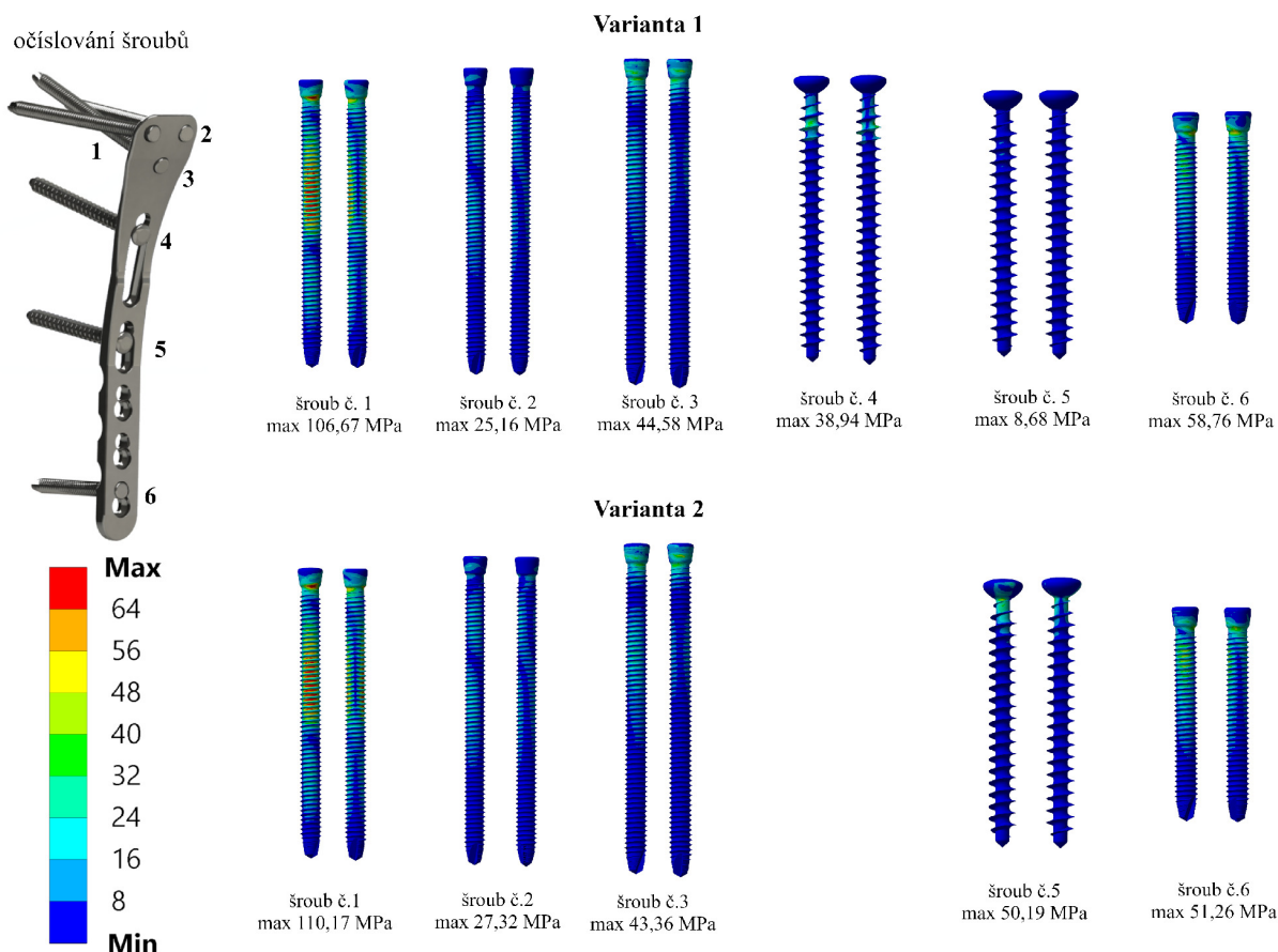
Obrázek 11.7: Redukované napětí HMH na šroubech pro Varianty 1 a 2 [MPa]
