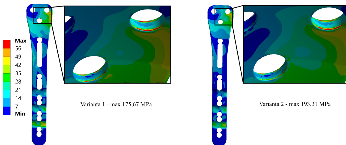
Obrázek 11.6: Maximální napětí na dlaze pro Varianty 1 a 2 - detail [MPa]
