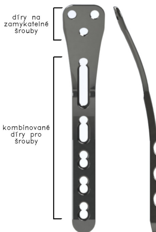
Obrázek 8.2: Dlahu pro fixaci zlomeniny postero-mediální části proximální tibie, vytvořeno na základě [1]
