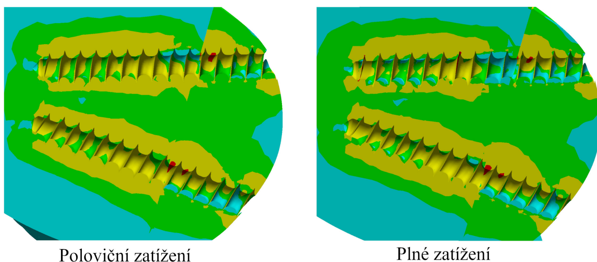
Obrázek 11.13: Redukované přetvoření HMH na spongiózní kostní tkáni zobrazené v řezu u Varianty 3 [-]
