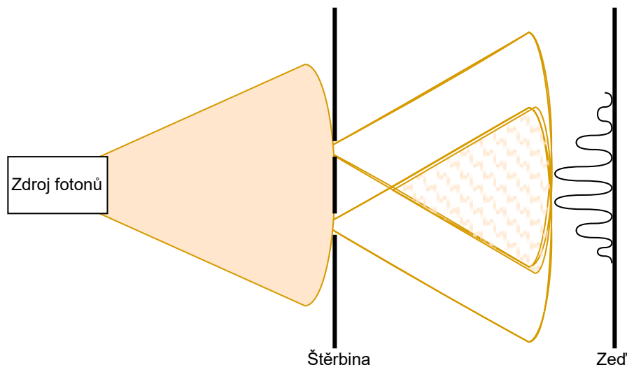
Obrázek 2.1: Youngův experiment
