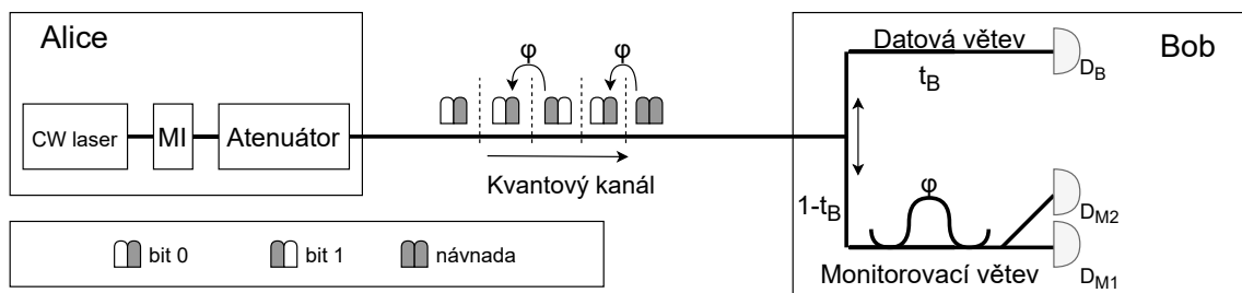
Obrázek 2.9: COW
