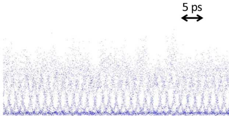
Obr. 3.40: Opticky navzorkovaný diagram oka 640Gbit PC-OTDM NRZ-OOO signálu po přenosu testovací trasou.
