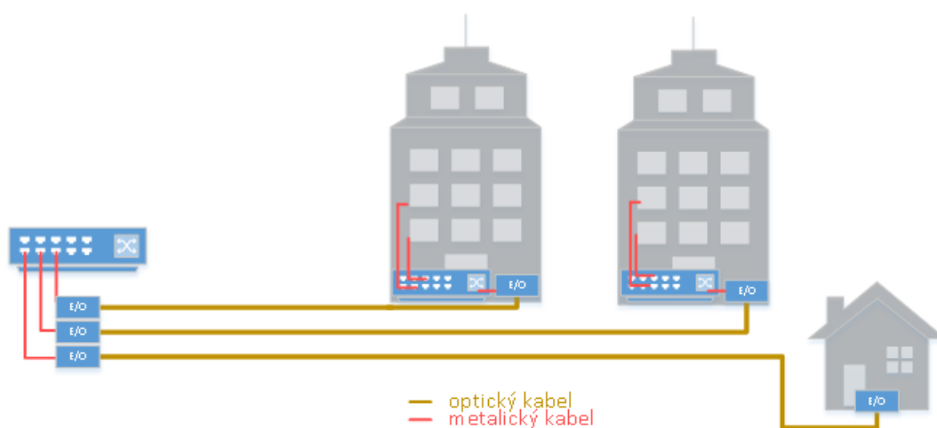
Obr. 3.20: Model sítě s použitím media-konvertorů.
