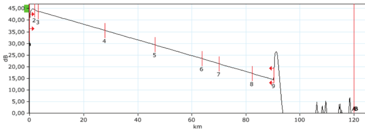
Obr. 3.15: OTDR průběh trasy 8 pro vlnovou délku 1 310 nm.
