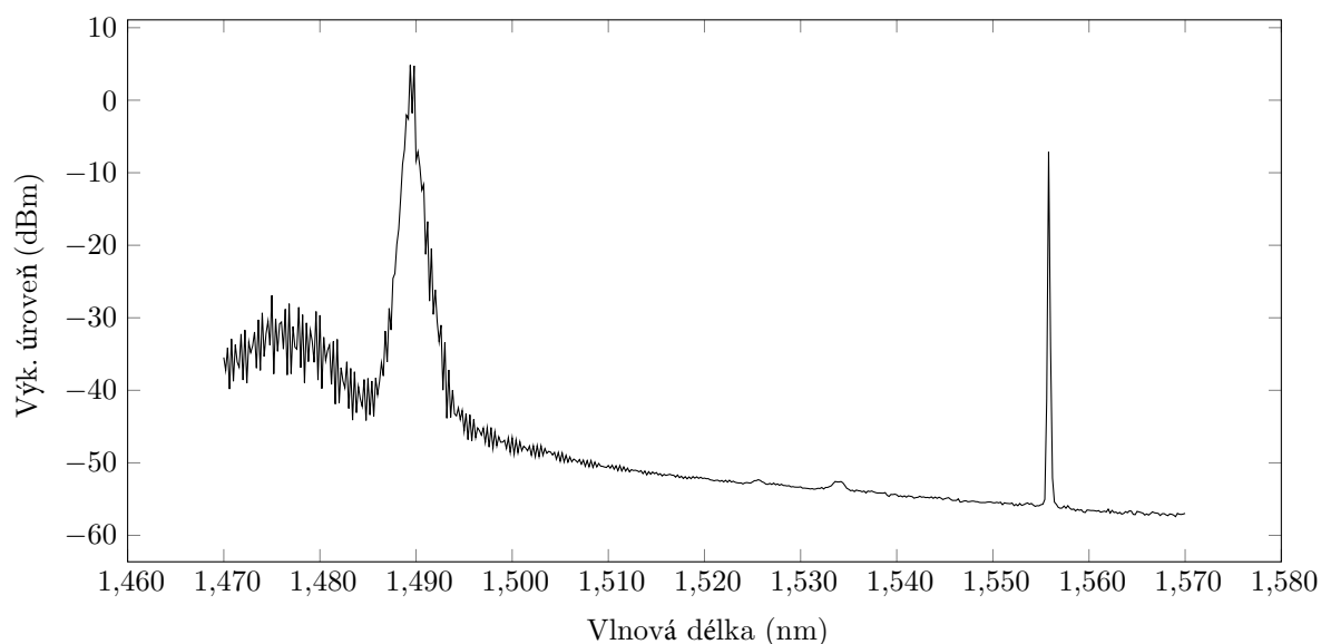
Obr. 3.57: Výstup OSA měřený za optickým rozbočovačem 2.
