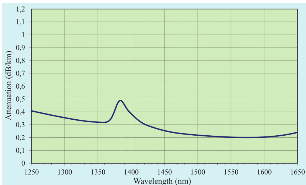
Obr. 3.16: Spektrální profil vlákna.
