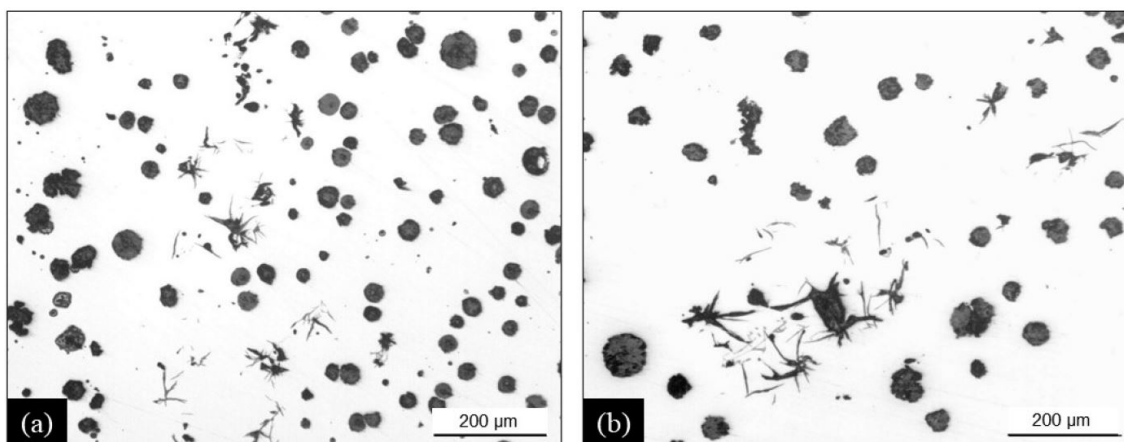
Obr. 21: Mikrostruktura vzorků s přidáním 0,004 hm. % Sb [25].
