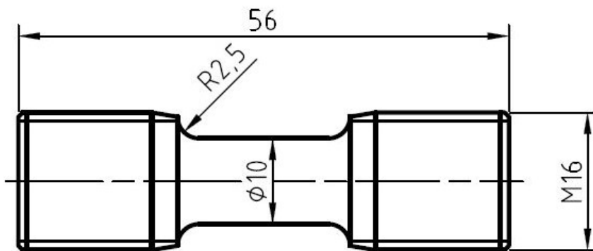
Obr. 24: Rozměry a tvar vzorků pro tahovou zkoušku.
