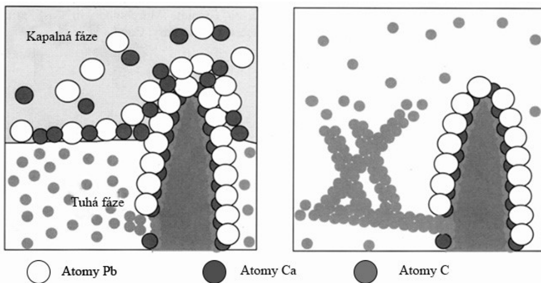
Obr. 4: Vznik Widmanstättenovy struktury grafitu [9].
