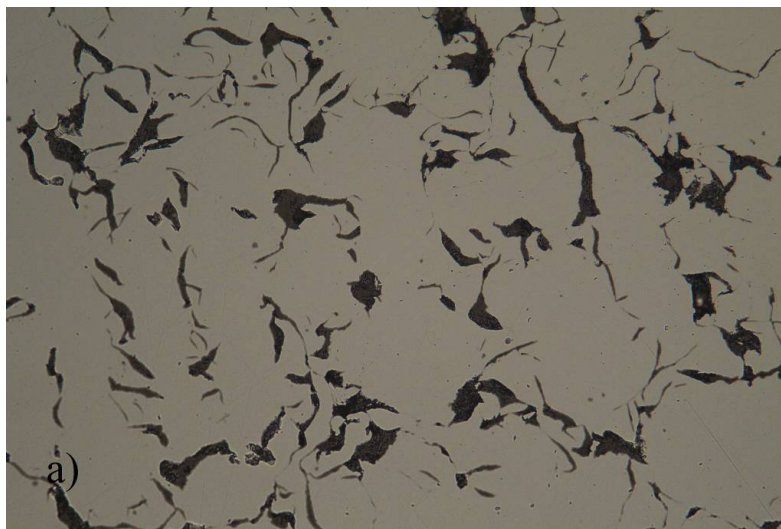
Obr. 32(a): Metallografický výbrus vzorku č. 6.
