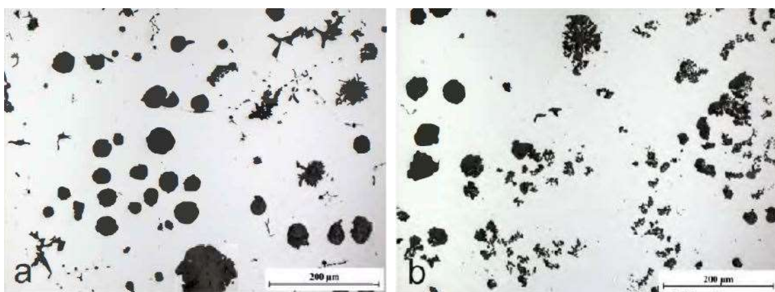
Obr. 17: Mikrostruktura s Pb (a) a mikrostruktura s Pb a Ce (b) [13].
