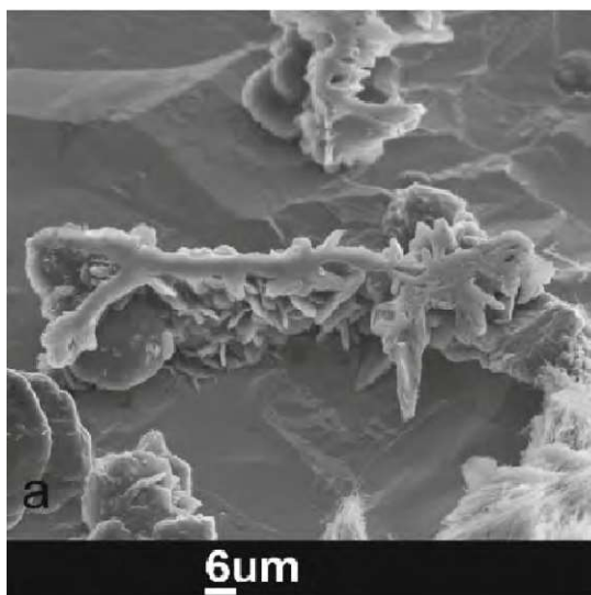
Obr. 18: Mikrostruktura vzorku s přebytkem Pb, grafitové lupínky a spiky grafit [13].
