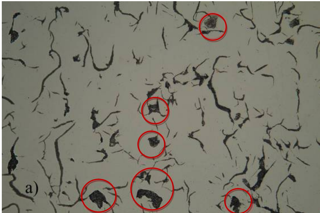
Obr. 28(a): Metalografický výbrus vzorku č. 2.
