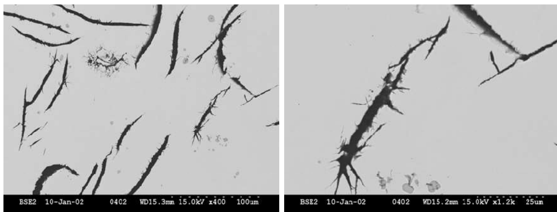
Obr. 5: Widmanstättenova struktura grafitu [10].
