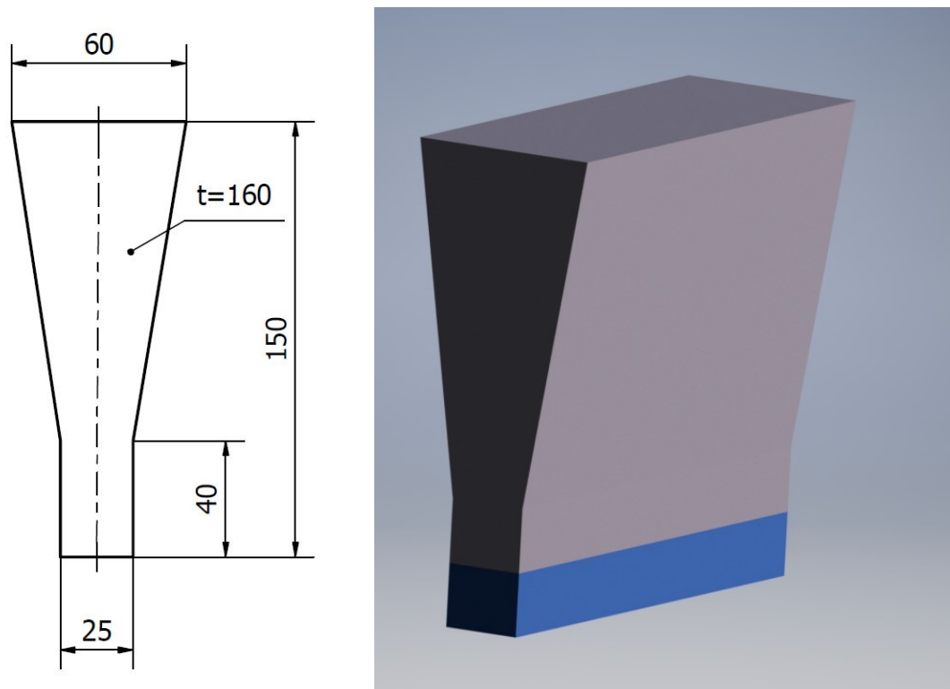
Obr. 23: Rozměry odlévaných bloků a místo odběru vzorků pro tahovou a útlumovou zkoušku.
