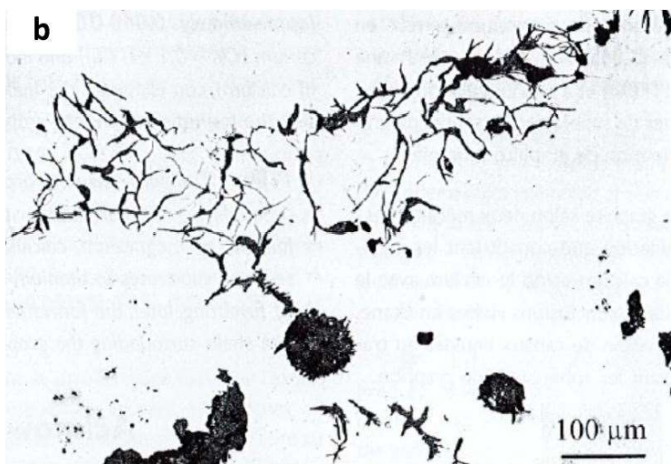
Obr. 12: Spiky grafit rozvětvený do síťového grafitu [19].
