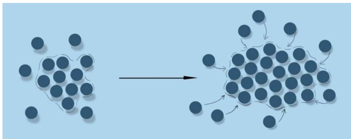
Obr. 3: Nukleace zárodků [7].
