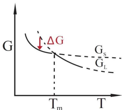
Obr. 2: Gibbsova energie [5].
