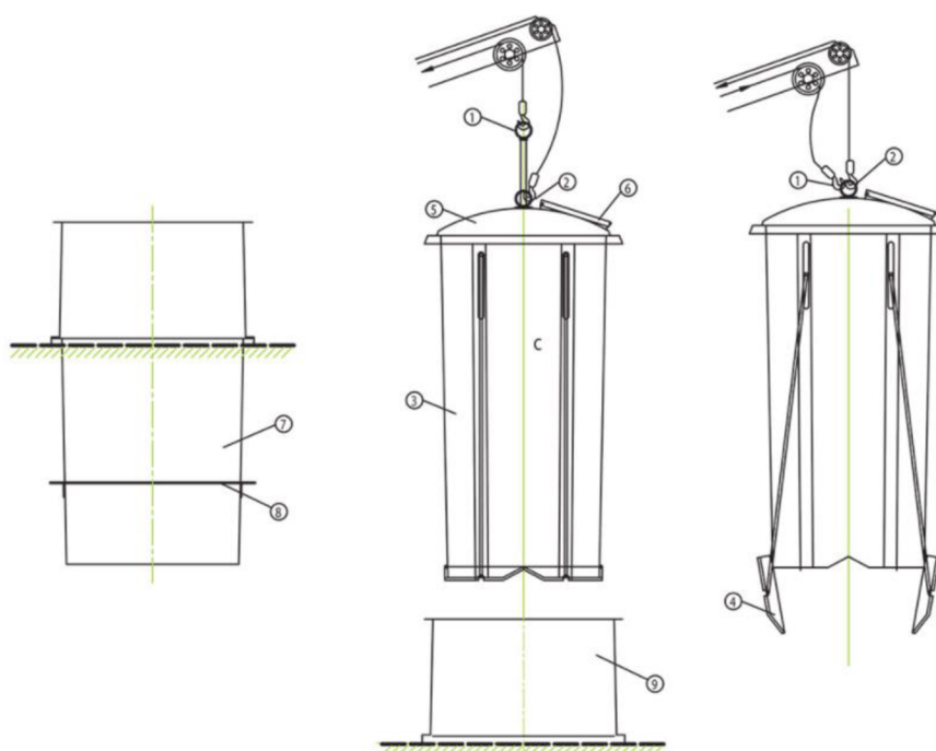
Obrázek 19 Schéma polopodzemního kontejneru, dostupné z: http://www.reflex-zlin.cz/podzemni-kontejnery-castecne-zapustene-semi/konstrukce-kontejneru/
