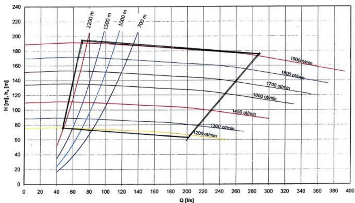
Obrázek 9: graf Q - H MČS 180/330K, křivky výtlaku pro 1 \times DN 150 různých délek [1]
