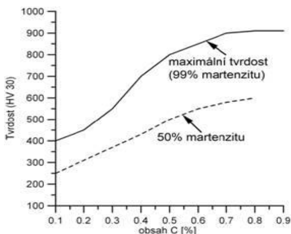
Obr. 2.1: Závislost tvrdosti oceli s 50 a 99,9% martenzitu na obsahu uhlíku [3].
