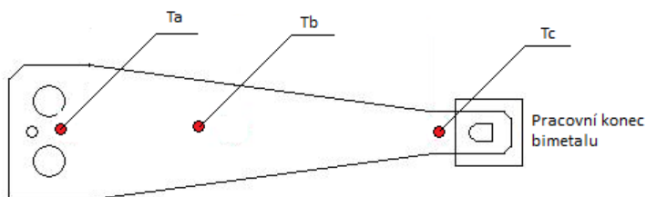
Obr. 27: Rozložení termočládku na pasivní vrstvě bimetalu Y1 pro měření teploty
