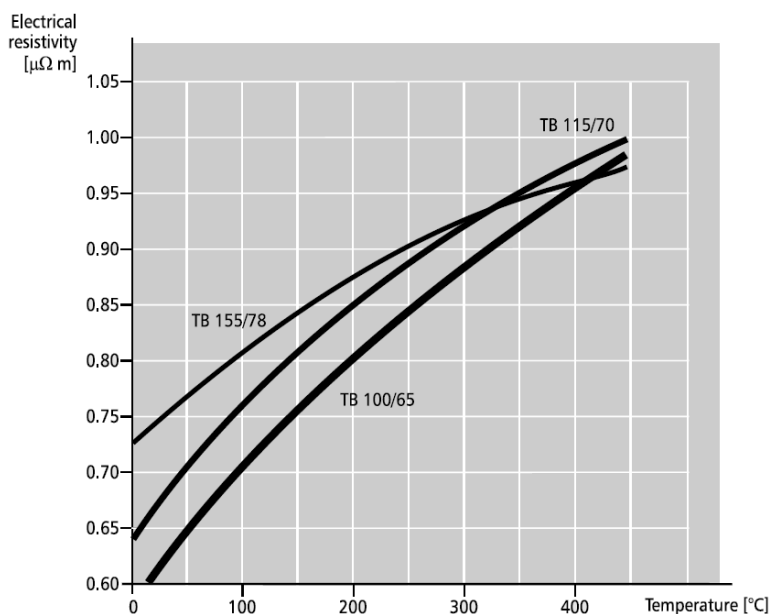
Obr. 14: Teplotní závislost měrného elektrického odporu pro různé typy bimetalu [2]
