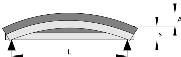
Obr. 8: Zakřivení prostě podepřeného bimetalového pásku [2]
