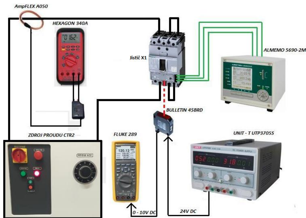
Obr. 28: Schéma zapojení pro měření volného průhybu
