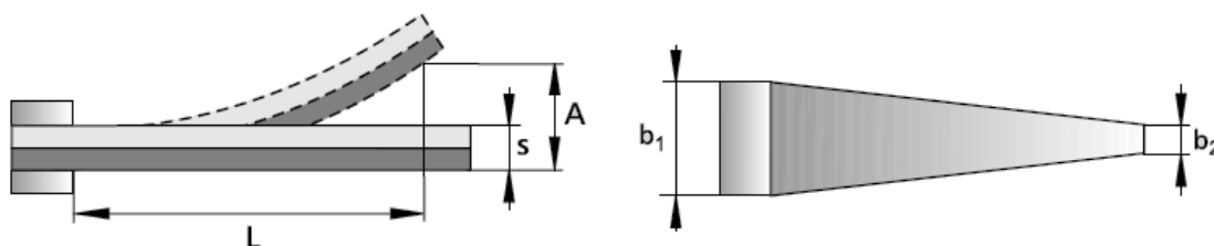
Obr. 19: Definice rozměrů jednostranně upevněného bimetalu zkoseného tvaru [2]
