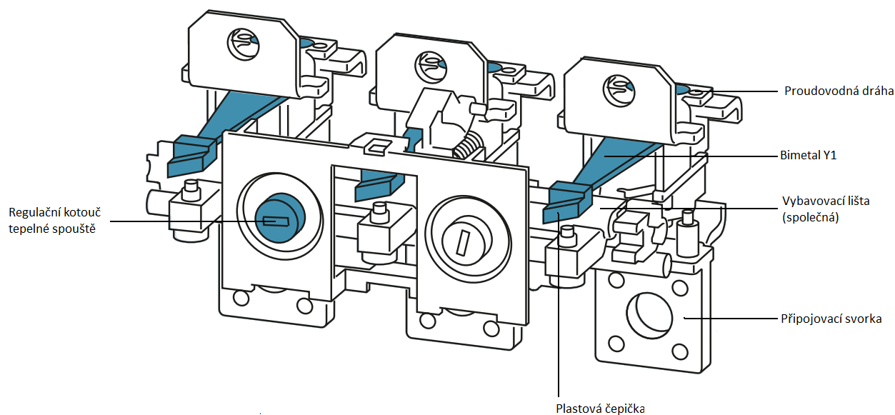
Obr. 22: Termomagnetická nadproudová spoušť jističe XI [9]
