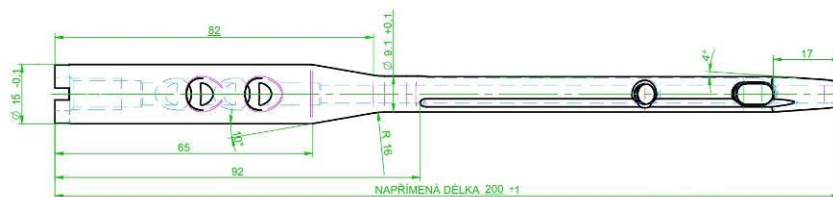
Obr. 6.1 Konstrukční návrh nitrodřeňového hřebu.
