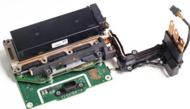
Obr. 8: Invertor elektromobilu.
