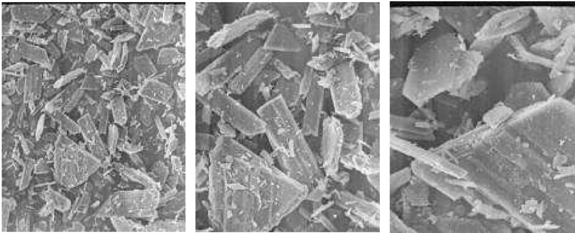
Obr 18: Morfologie sádrovce TR Pregips zachycená REM
