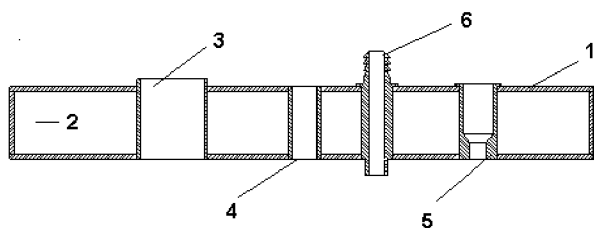
Obr 24: Řez víkem
