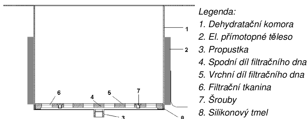
Obr 23: Schéma dehydratační komory
