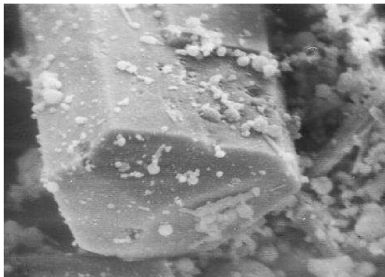
Obr 4: \alpha -sádra ve formě automorfních zrn bassanitu (hemihydrátu) (zvětšení 4000x)
