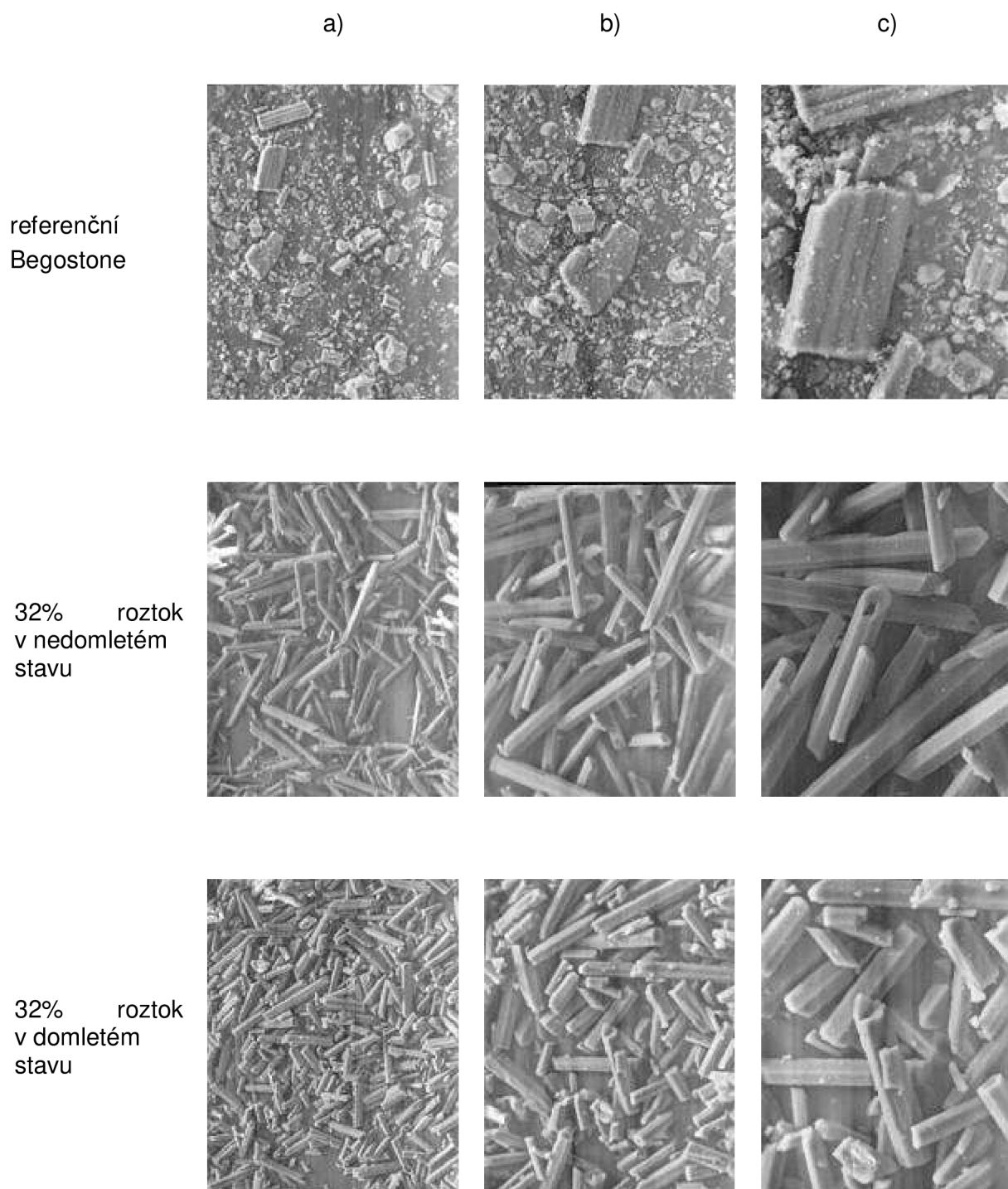
Obr 90: Morfologie sádry připravené v dehydratačním roztoku \text{CaCl}_2 o koncentraci 32% v nedomletém a domletém stavu při zvětšení a) 300x, b) 600x, c) 1200x
