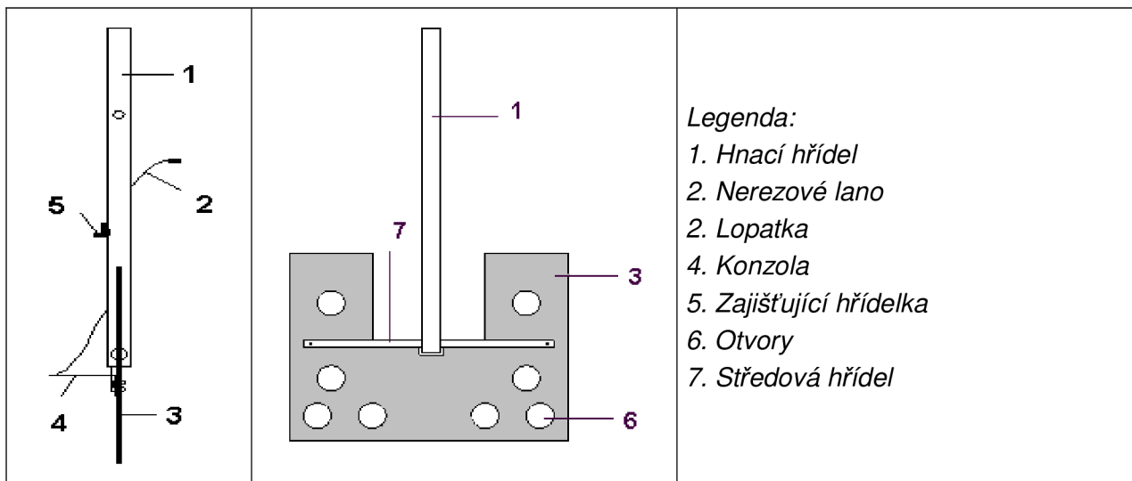
Obr 25: Schéma míchadla
