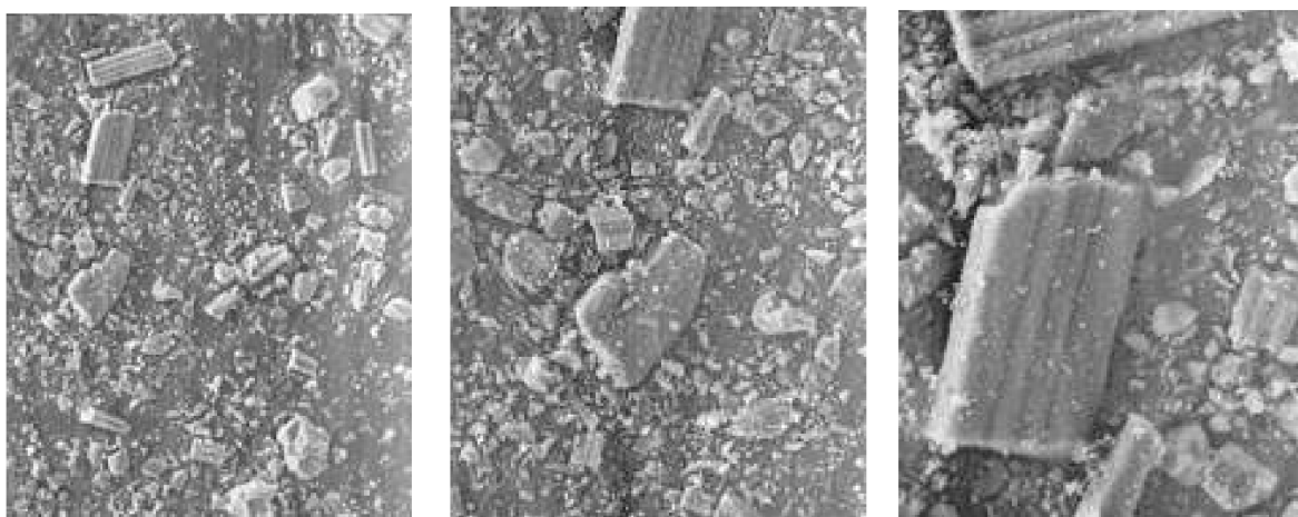
Obr 20: Morfologie referenční sádry Begostone při zvětšení
