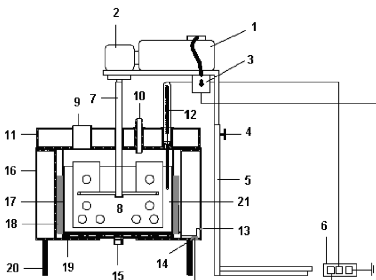
Obr 22: Schéma jednokomorového dehydrátoru
