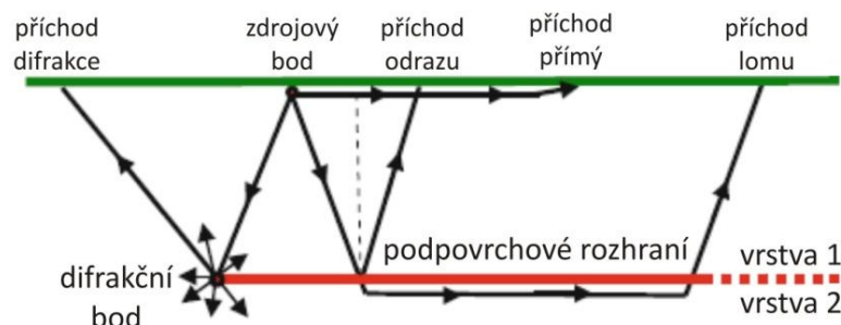
Obr. 18: Čtyři typy příchozích vln, které jsou nejčastěji zaznamenány (Alsadi 2017).
