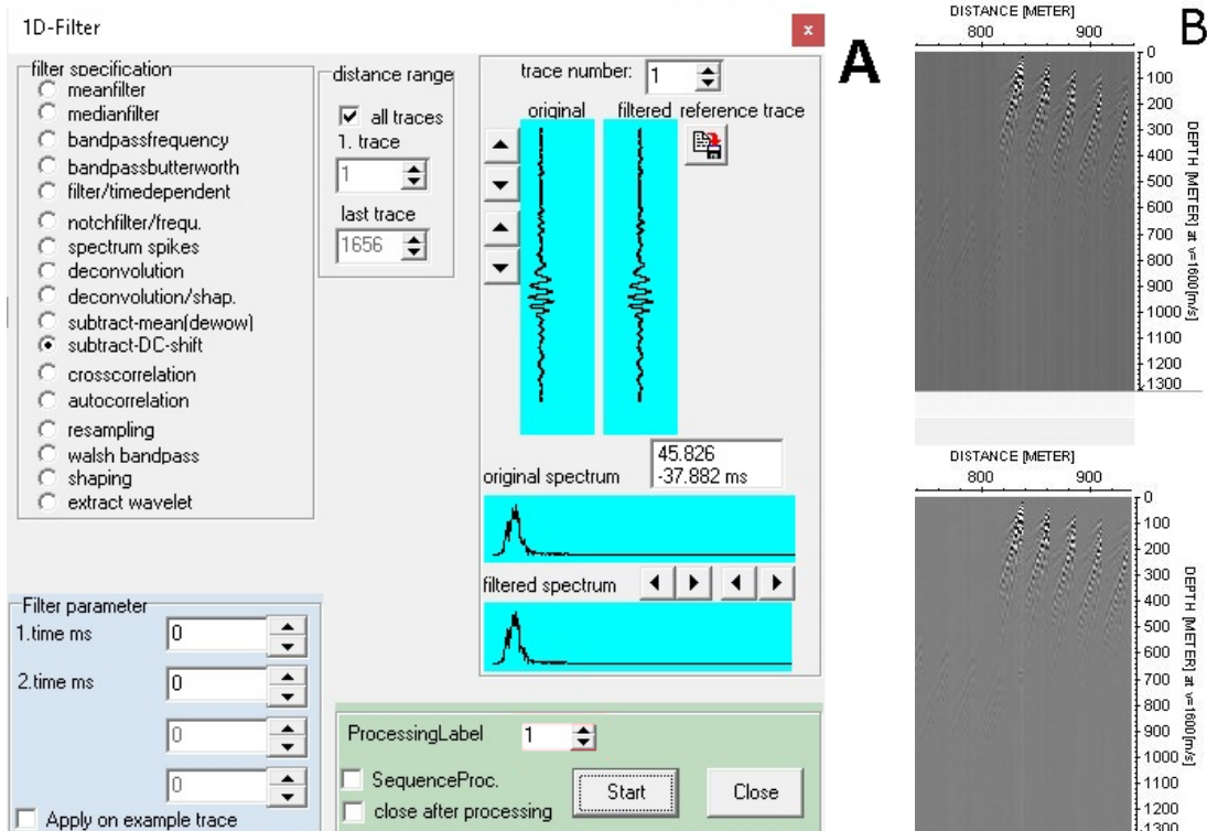
Obr. 29: Subtract-DC-shift; A) zadávání jednotlivých parametrů; B) profil před (nahore) a po (dole) filtračním kroku.
