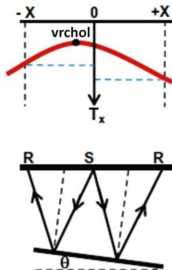
Obr. 21: NMO koncept v případě klesajícího reflektoru (Alsadi 2017).
