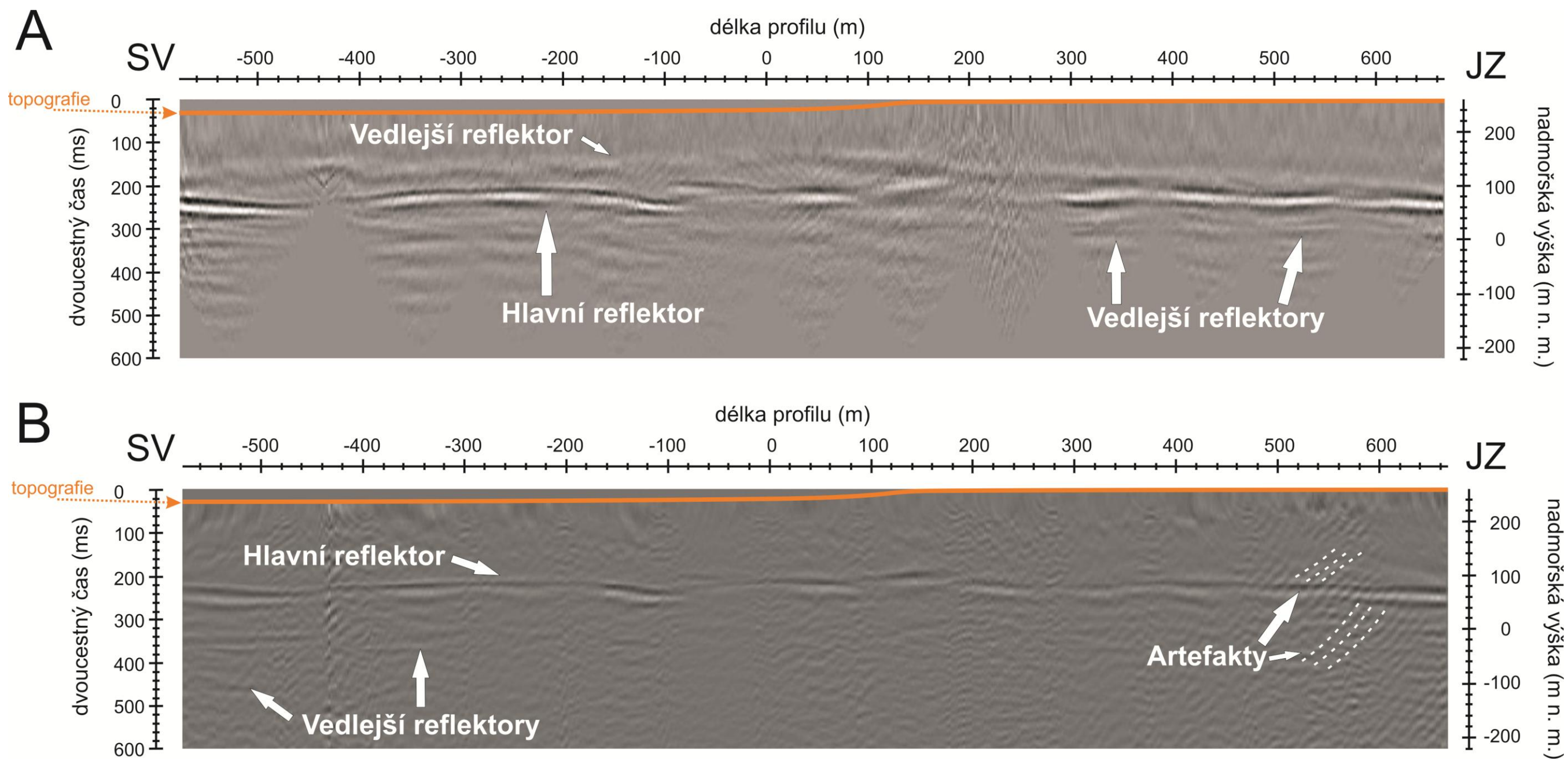
Obr. 44: Profil Držovice stackovaný při rychlostní analýze; A) při použití filtračního kroku muting; B) při použití filtračního kroku fk filtr-lineparts.
