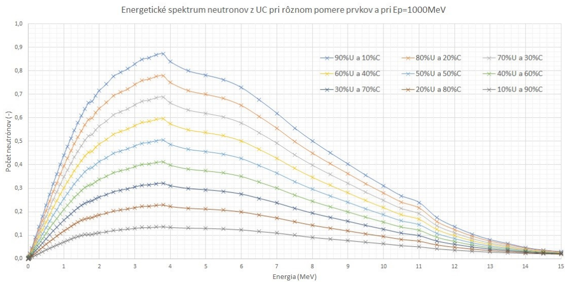
Obr. C.9: Energetické spektrum neutrónov pre rôzne pomery uránu v zlučénine UC
