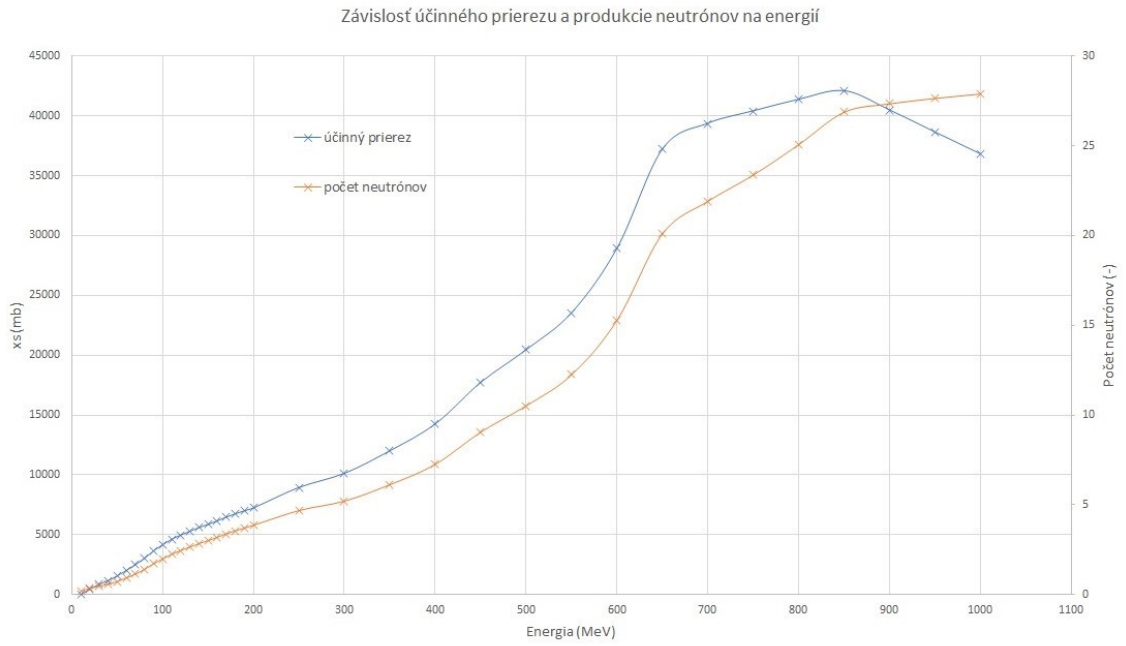
Obr. C.1: Závislosť účinného prierezu a produkcie neutrónov na energií protónu pre prírodnú zmes uránu
