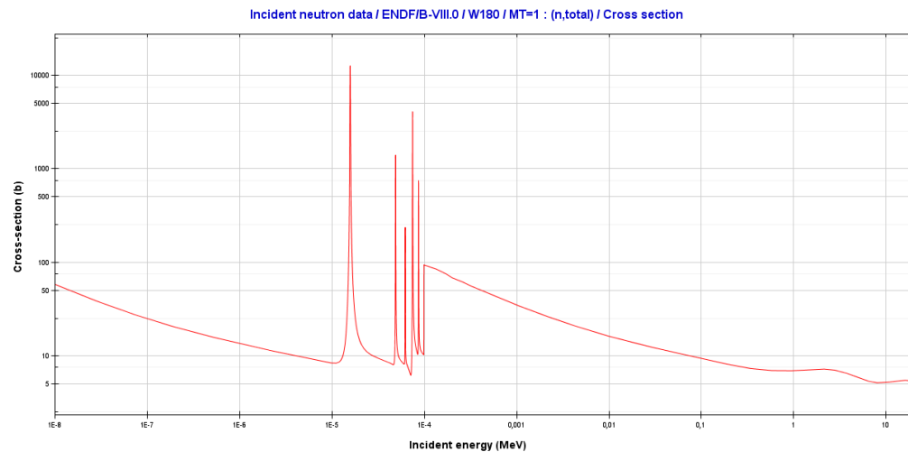
Obr. B.4: Účinný prierez ^{180}\text{W} v závislosti na energií neutrónu [25]
