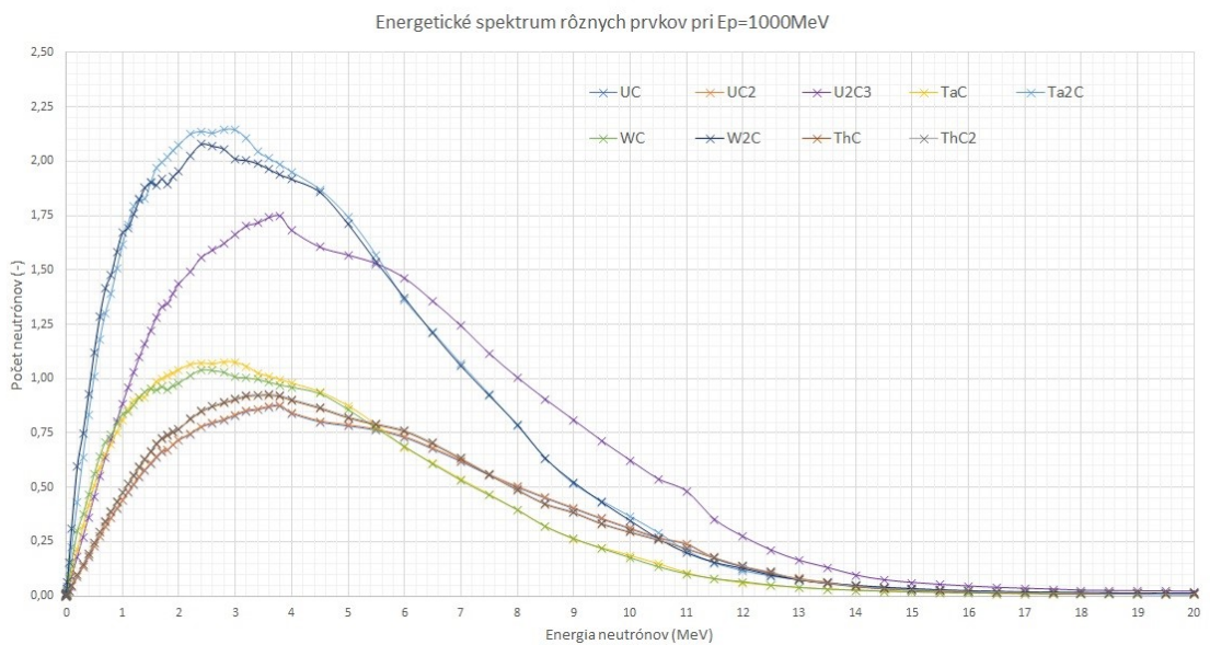
Obr. C.10: Energetické spektrum neutrónov pre rôzne zlučéniny s pomerom 90% ťažký prvok a 10%C
