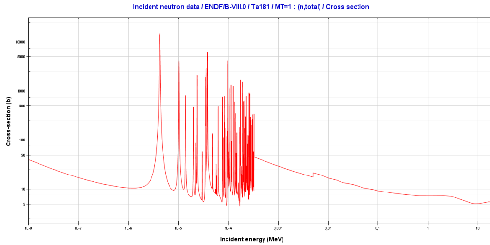
Obr. B.3: Účinný prierez ^{181}\text{Ta} v závislosti na energií neutrónu [25]
