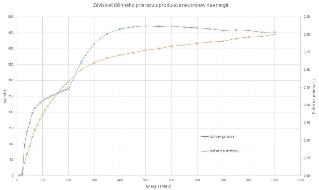
Obr. C.2: Závislosť účinného prierezu a produkcie neutrónov na energií protónu pre prírodnú zmes uhlíku
