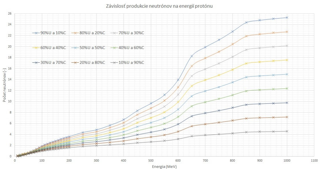
Obr. C.4: Závislosť produkcie neutrónov na energií protónu pre rôzne pomery uránu v zlučene UC
