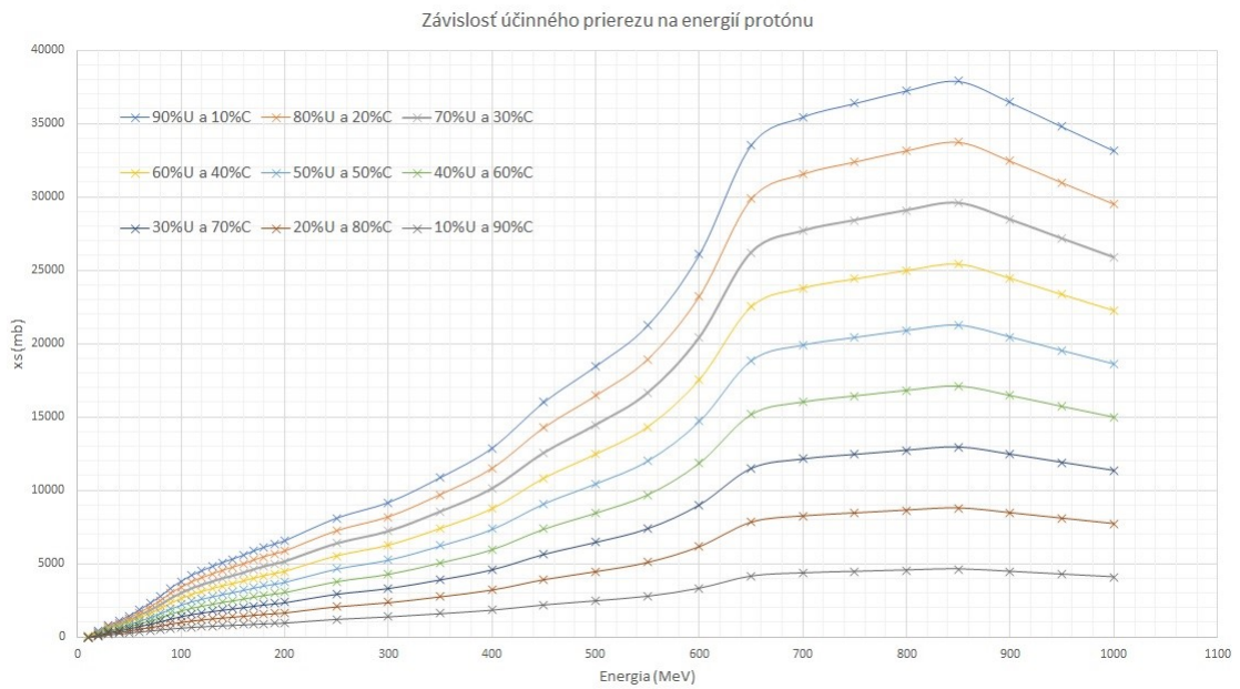
Obr. C.3: Závislosť účinného prierezu na energií protónu pre rôzne pomery uránu v zlučene UC
