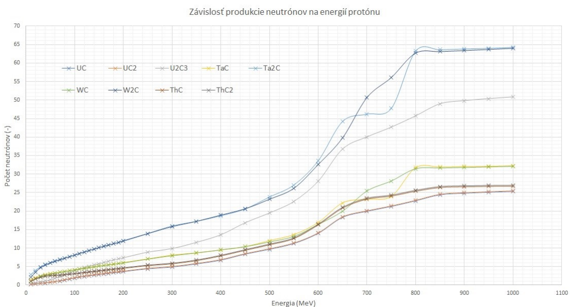
Obr. C.6: Závislosť produkcie neutrónov na energii protónu pre rôzne zlúčeniny s pomerom 90% ťažký prvok a 10%C
