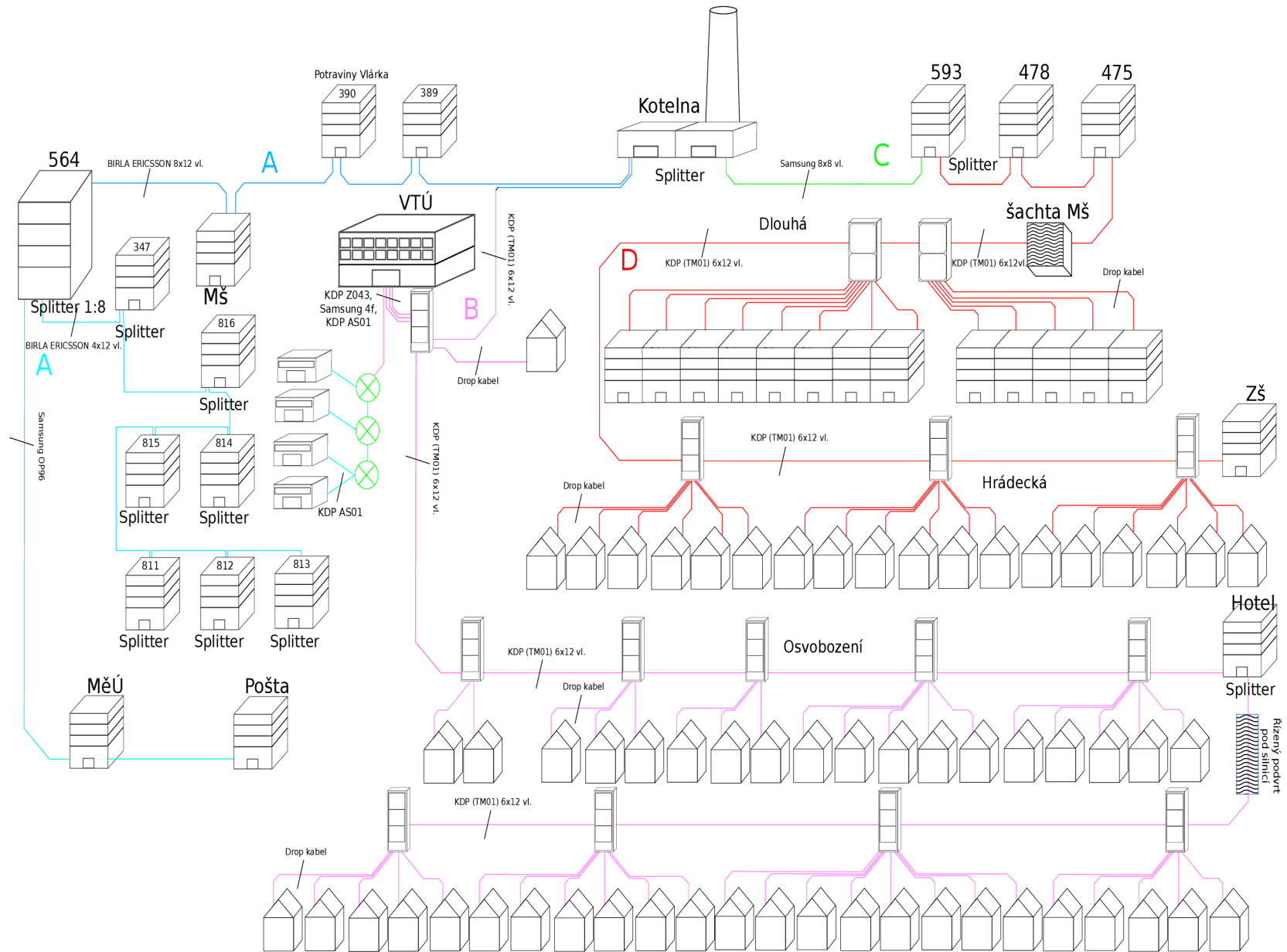
Obr. D.2: Schéma použití kabelů na trasách
