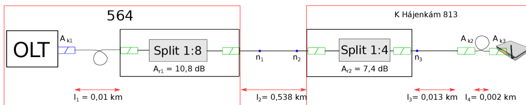
Obr. 7.7: Topologie nejvzdálenější přípojky na trase A.
