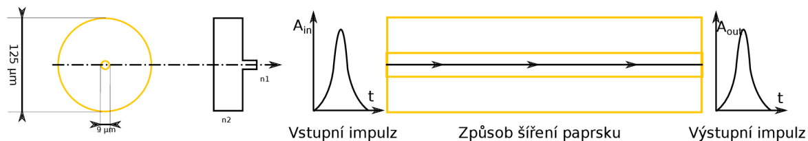
Obr. 1.4: Jednovidové vlákno[1]
