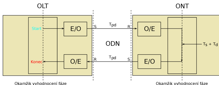
Obr. 5.2: Grafické znázornění jednotlivých zpoždění[17]
