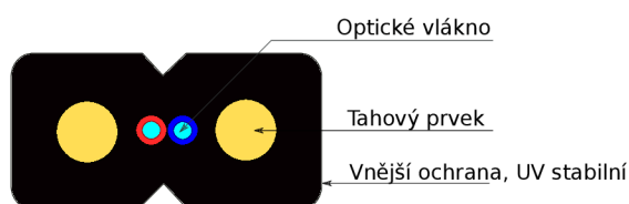
Obr. 6.12: Příčný řez optickým kabelem FLAT DROP FRP 2F (Z043)[27]
