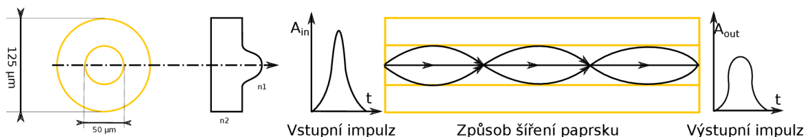
Obr. 1.3: Mnohavidové vlákno s gradientní změnou indexu lomu[1]
