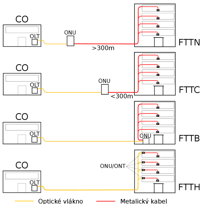
Obr. 3.1: Grafické znázornění čtyř základních konfigurací FTTx[5]
