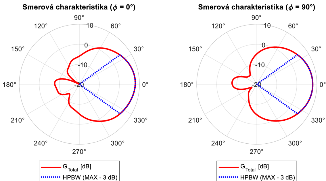
Obr. 34: Smerové charakteristiky zisku fľačkovej antény vyklopenej okolo hrany kostry satelitu
