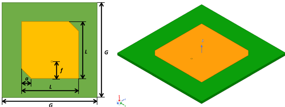
Obr. 20: Výsledná podoba modelu navrhnujetej fliačkovej antény v programe ANSYS HFSS
