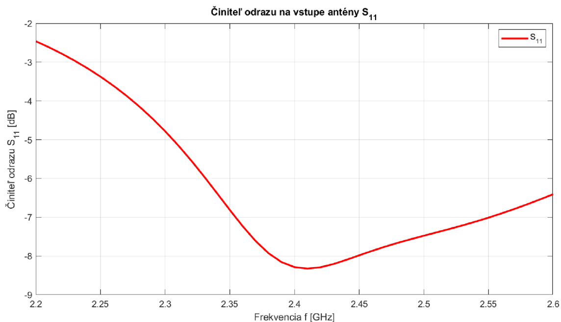
Obr. 51: Frekvenčná charakteristika činiteľu odrazu antény QFH v umiestnení nad rohom kostry satelitu
