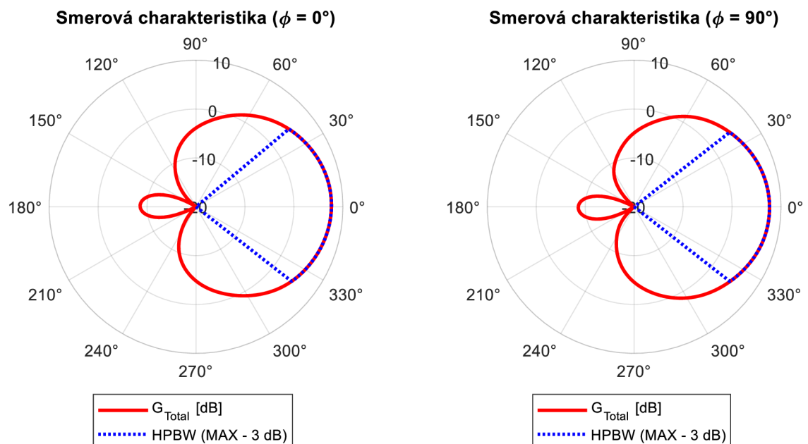
Obr. 21: Smerové charakteristiky zisku samotnej fliačkovej antény
