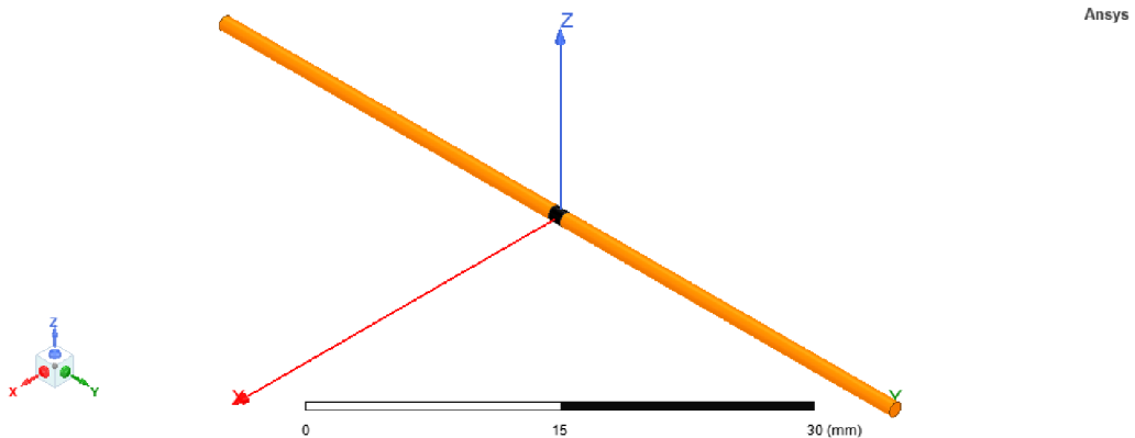
Obr. 8: Výsledná podoba modelu navrhnujej polvlnnej dipólovej antény
