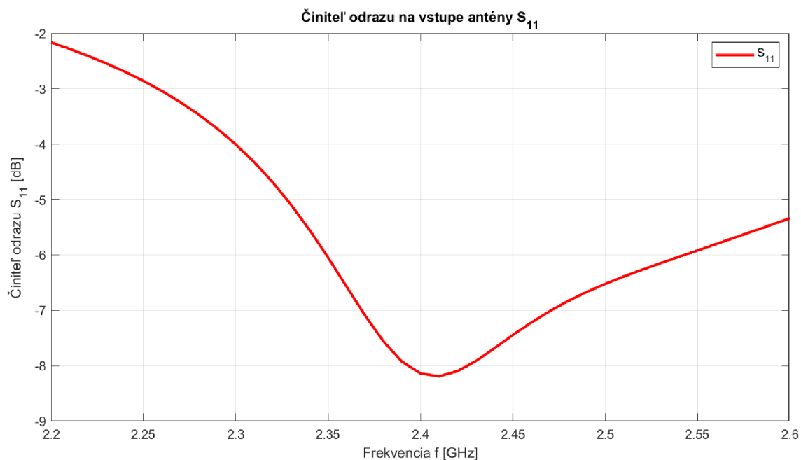
Obr. 43: Frekvenčná charakteristika činiteľu odrazu antény QFH v umiestnení nad stredom steny kostry satelitu
