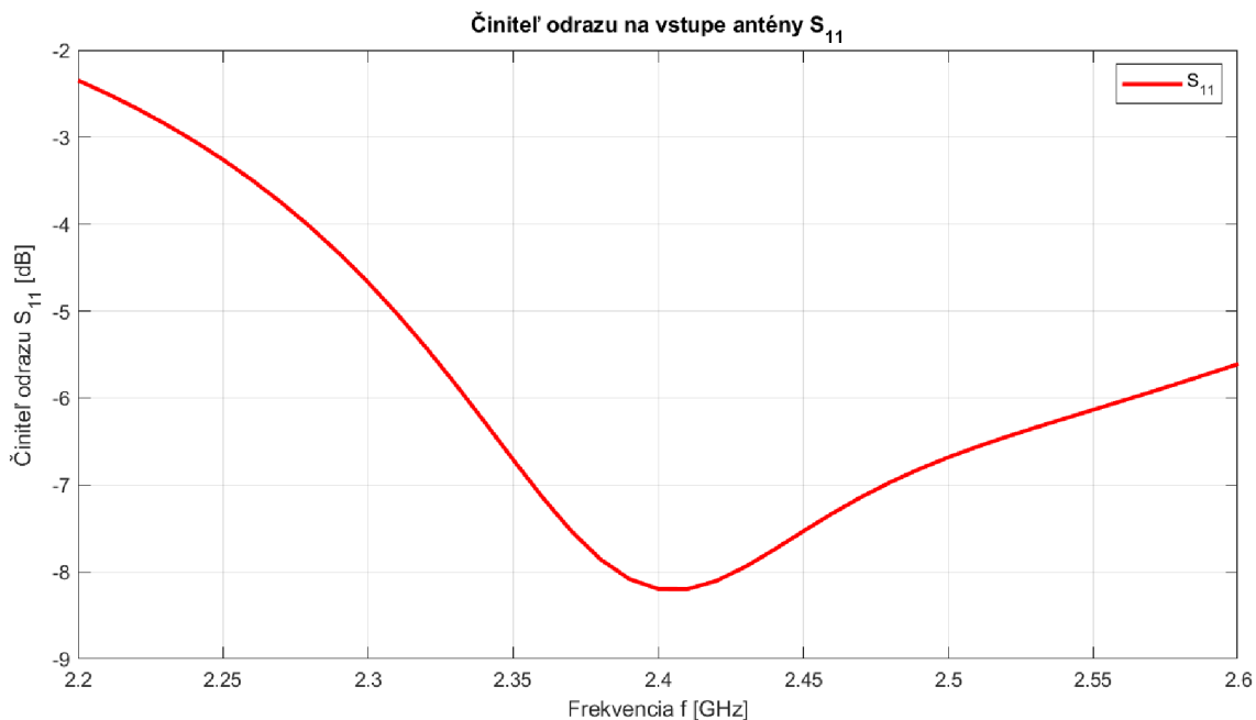
Obr. 47: Frekvenčná charakteristika činiteľu odrazu antény QFH v umiestnení nad stredom hrany kostry satelitu
