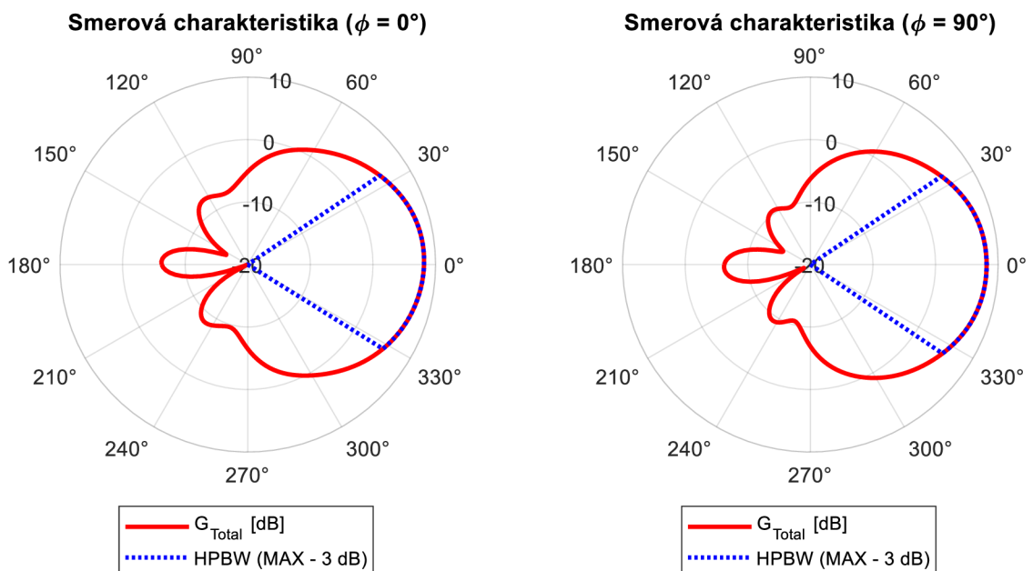
Obr. 25: Smerové charakteristiky zisku fliáčkovej antény v umiestnení v strede steny kostry satelitu
