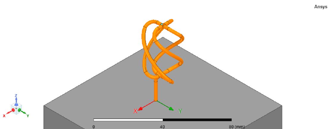
Obr. 53: Umiestnenie modifikovaného modelu antény QFH nad stredom steny kostry satelitu
