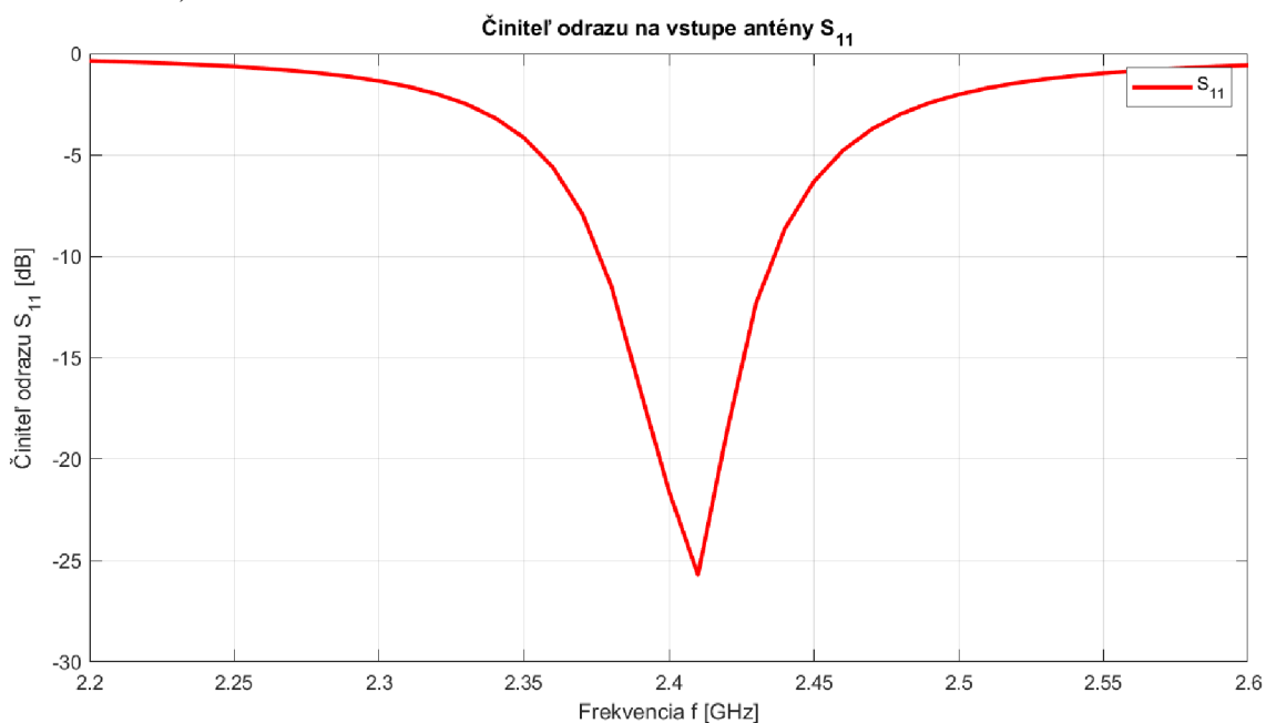
Obr. 35: Frekvenčná charakteristika činiteľu odrazu fľačkovej antény vyklopenej okolo hrany kostry satelitu
