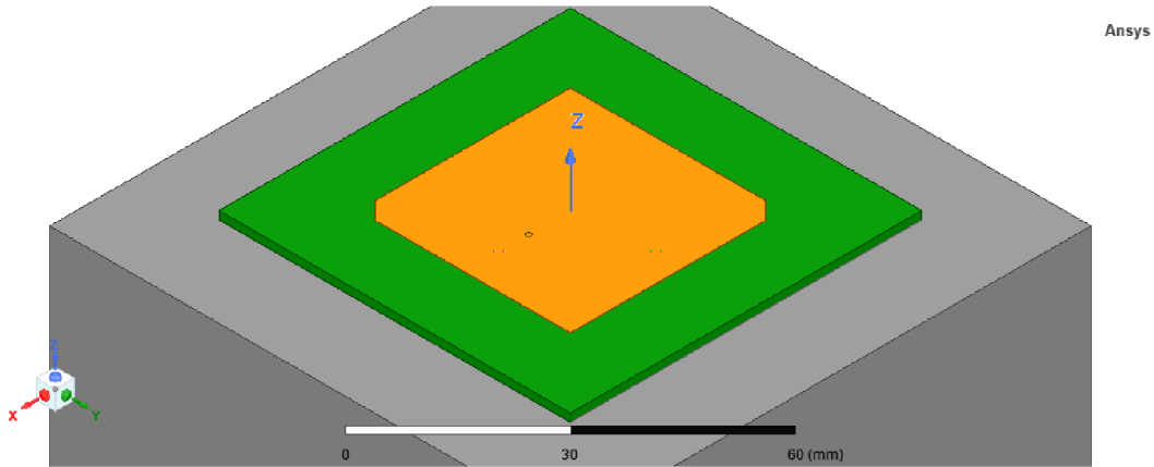
Obr. 24: Umiestnenie fliáčkovej antény v strede steny kostry satelitu
