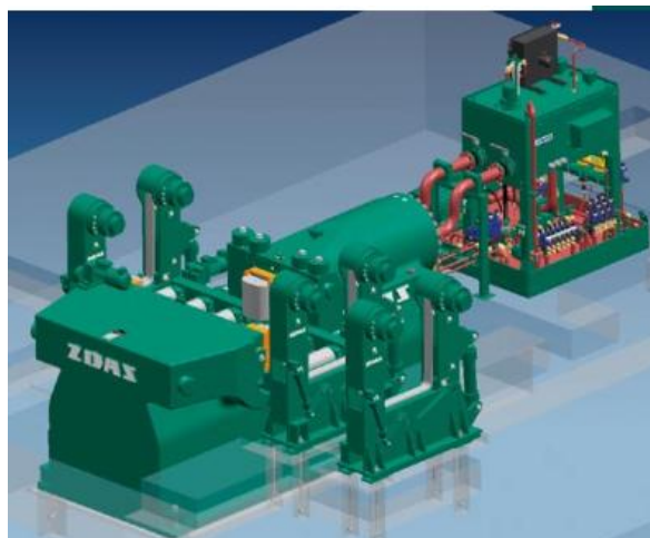
Obr. 6: Rovnací lis na tyčový materiál ŽDAS CDT 1000[9]
