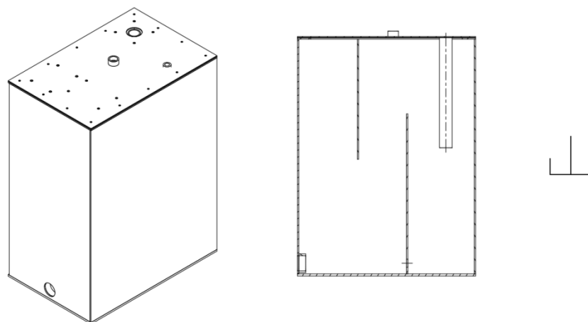
Obr. 13: Vějšší pohled na nádrž, uzpořádání přepážek a schématická značka nádrže.
