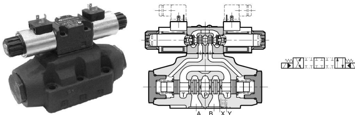
Obr. 16: Zvolený rozvaděč, jeho vnitřní uspořádání a schématická značka.[5]
