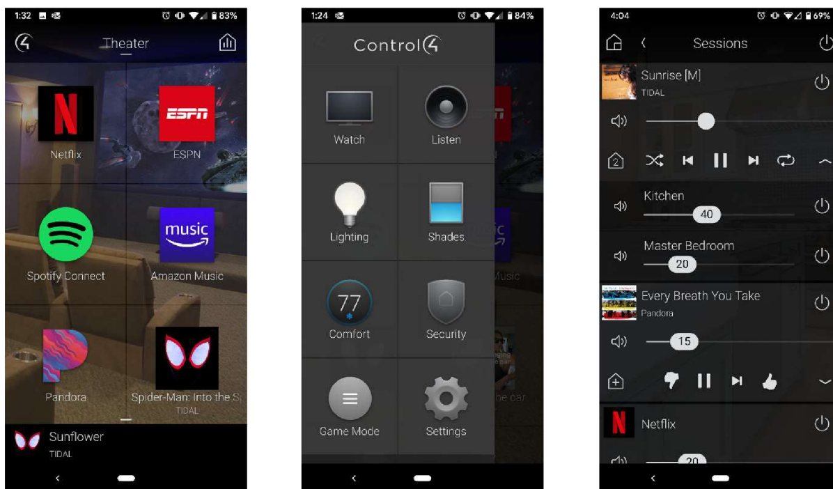
Obrázek 3.12 Aplikace Control4 [71]
