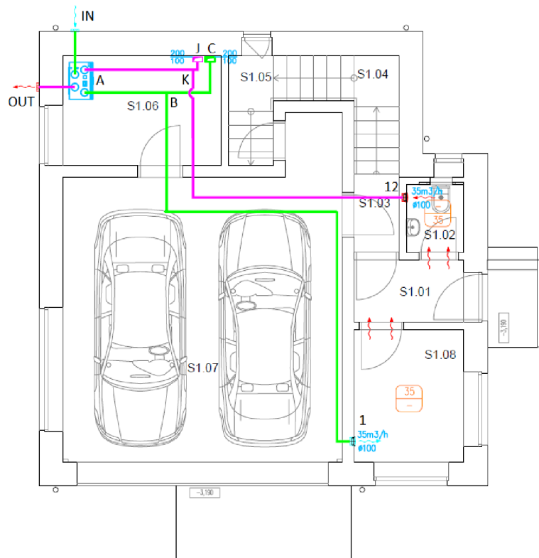
Obr. 3.4 – 1. PP schéma potrubní sítě (varianta č. 2)
