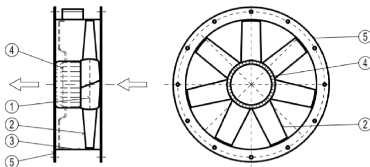
Obr. 1.4 – Axiální ventilátor [9]
