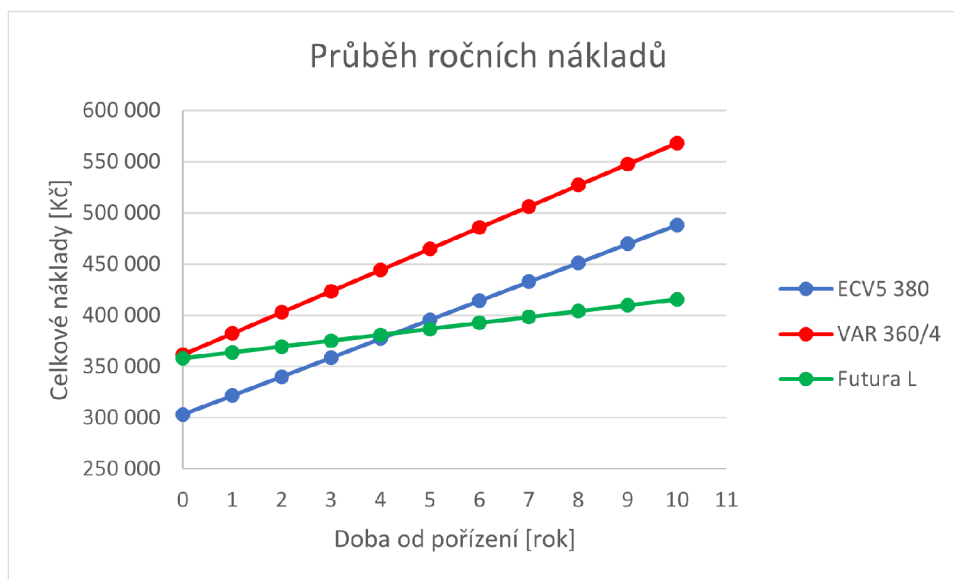
Obr. 4.1 – Průběh ročních nákladů
