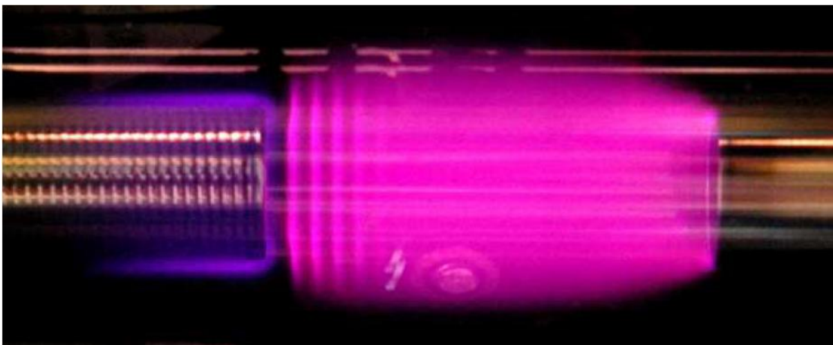
Obr. 2.4.2: Fotografie vrstevnaté struktury kladného světla (fotografie pořizená v laboratoři Plazmochemie na FCH VUT v Brně)
