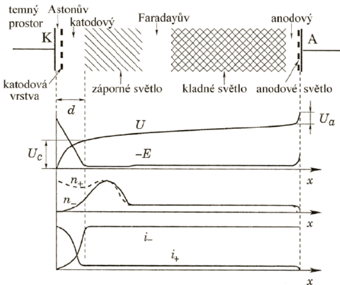
Obr. 2.4.1: Struktura doutnavého výboje a průběhy podélného elektrického pole E , potenciálu U , koncentrace nabitých částic n^+ a n^- a hustoty proudů kladných iontů a elektronů i^+ a i^- [8]
