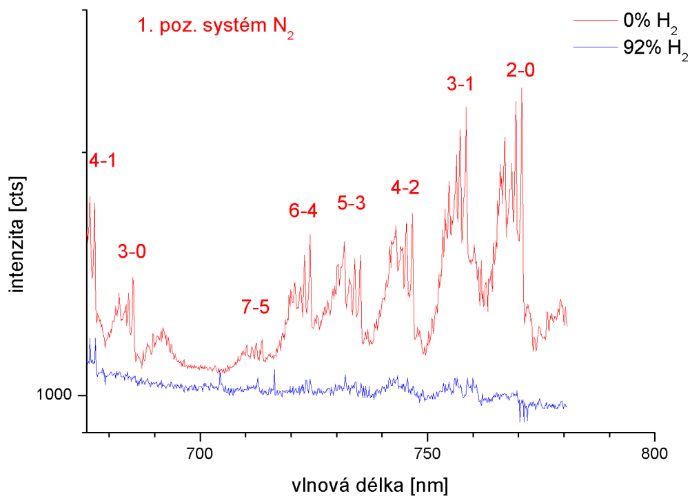
Obr. 4.1.4: Identifikované spektrum v rozsahu 675–780 nm v čase dohasínání 4,7 ms. Spektrum čistého dusíku bylo pořízeno s integrační dobou 3 s, spektrum ve směsi obsahující 92% vodíku s integrační dobou 180 s.
