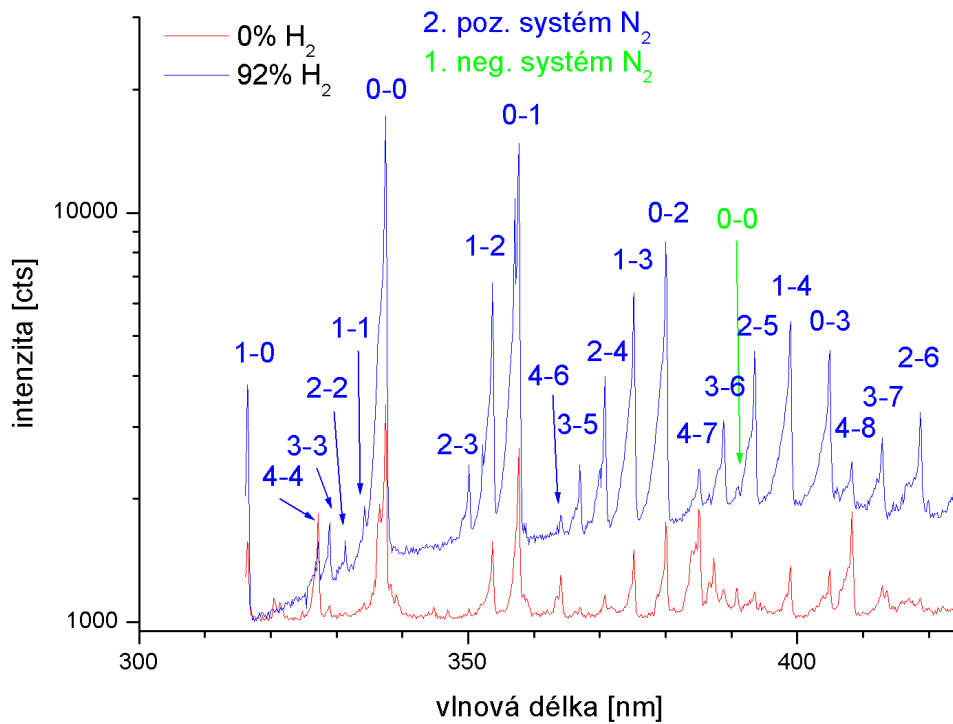
Obr. 4.2.1: Identifikované spektrum v rozsahu 316 – 425 nm v čase dohasínání 23,9 ms. Spektrum čistého dusíku bylo pořízeno s integrační dobou 3 s, spektrum ve směsi obsahující 92% vodíku s integrační dobou 60 s.
