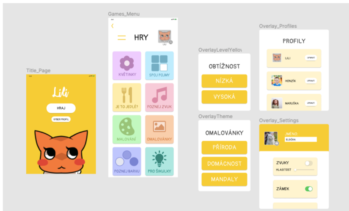
Vybraný návrh GUI
