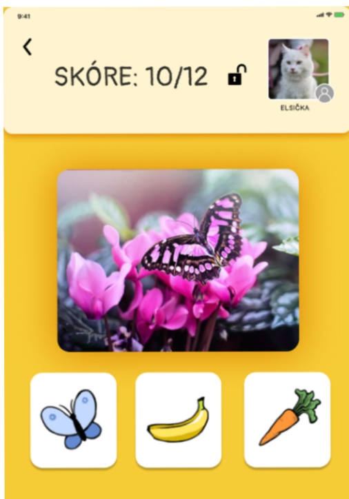
Hra pexeso
