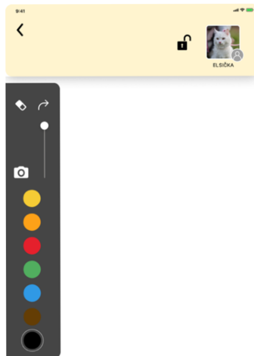
Hra malování
