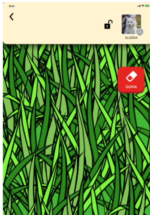
Hra kytičky
