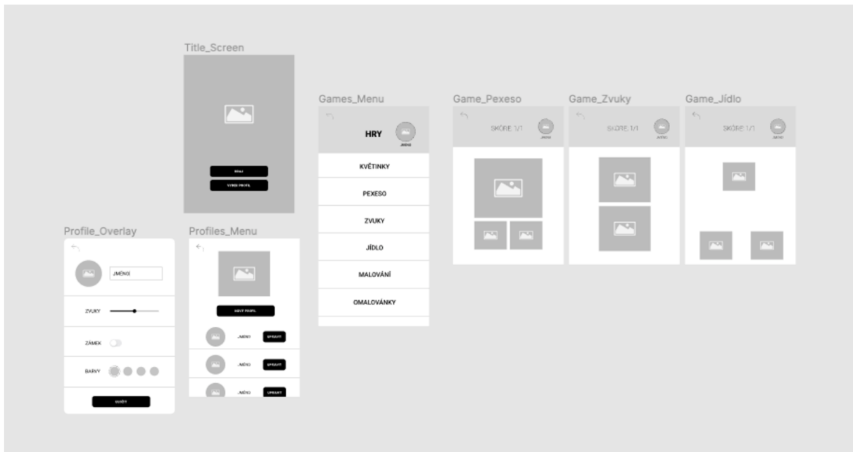
Vybraný wireframe
